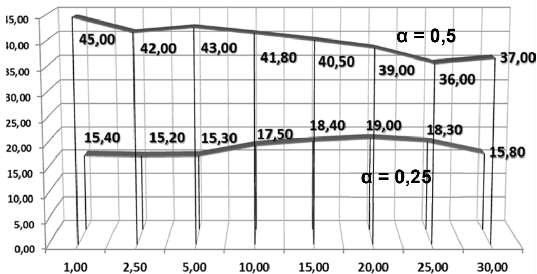
Рисунок 8 – Графики зависимости погрешности в определении угла крена судна по расчету и по программе COLOS от начального угла крена судна
