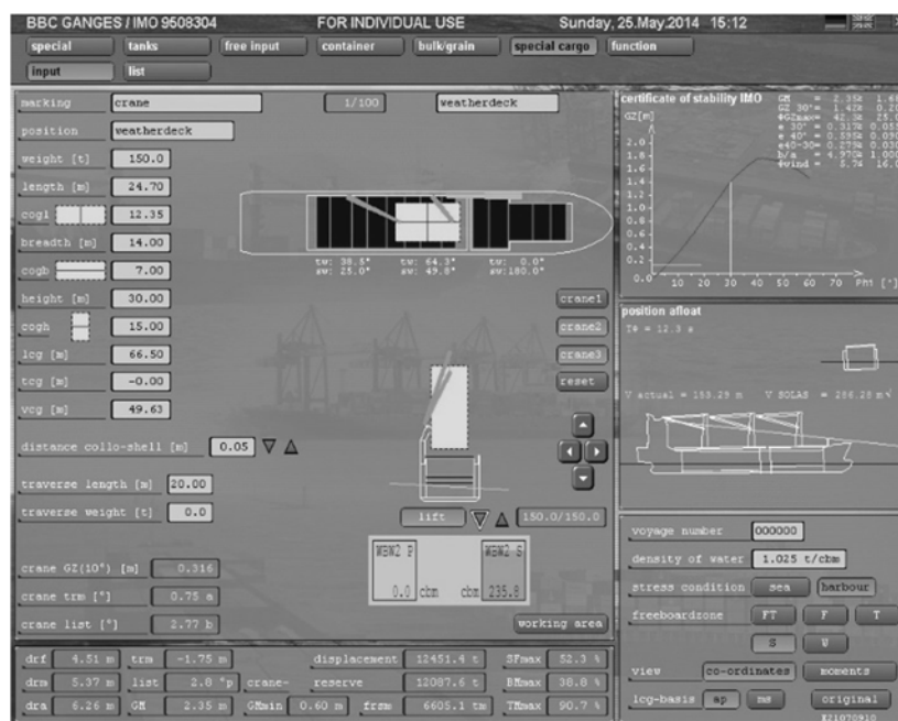
Рисунок 4 –Компьютерные расчеты в программе COLOS
