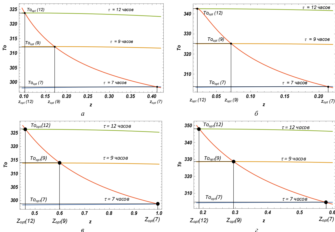
Рисунок 6 – Зависимость оптимальной доли неостекленных СК в составе двухкаскадной СВУ рассчитанная по распределенным параметрам:
