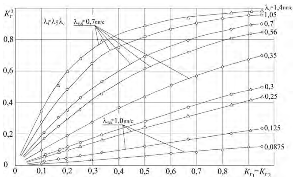
Рисунок 4 – Влияние величины коэффициента K_{Г1} = K_{Г2} готовности ЕТО 1 и ЕТО 2 на коэффициент K_{Г^3} готовности ЕТО 3 , состоящей из 2-х параллельных ЕТО i
