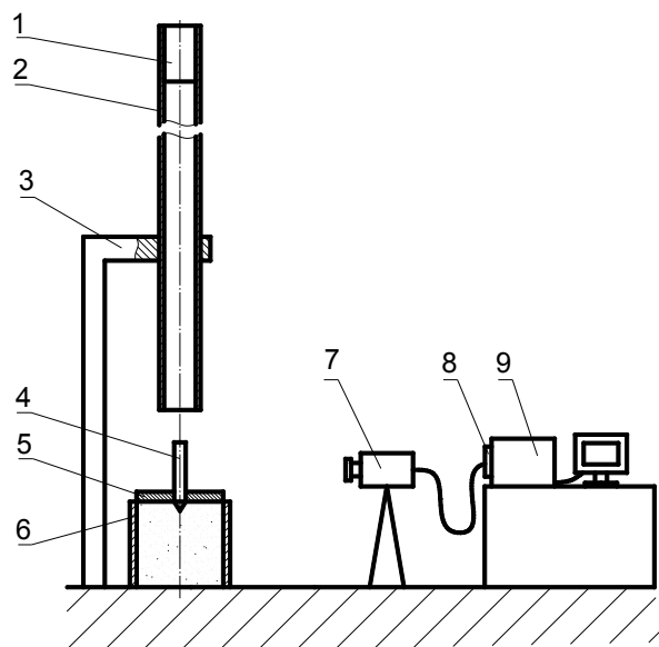
Рисунок 2 – Принципиальная схема экспериментальной установки:
