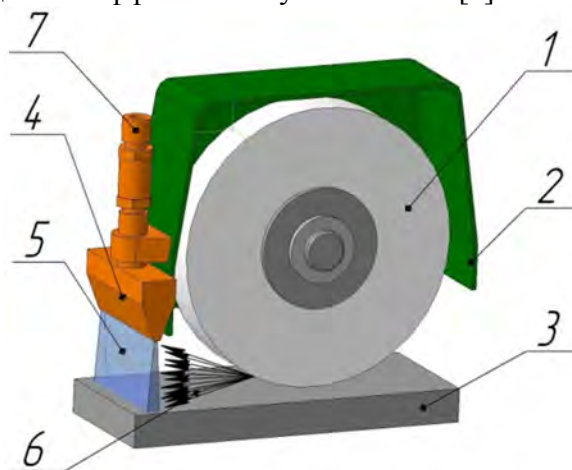
Рисунок 1 – Устройство заградительного способа подачи СОЖ:
