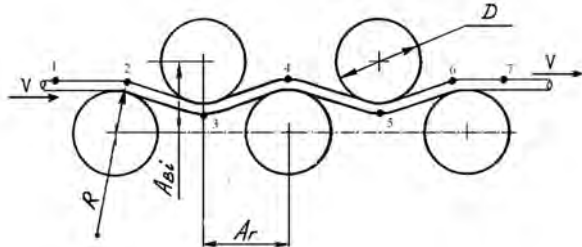
Рисунок 1 – Общая функциональная схема рихтователя
