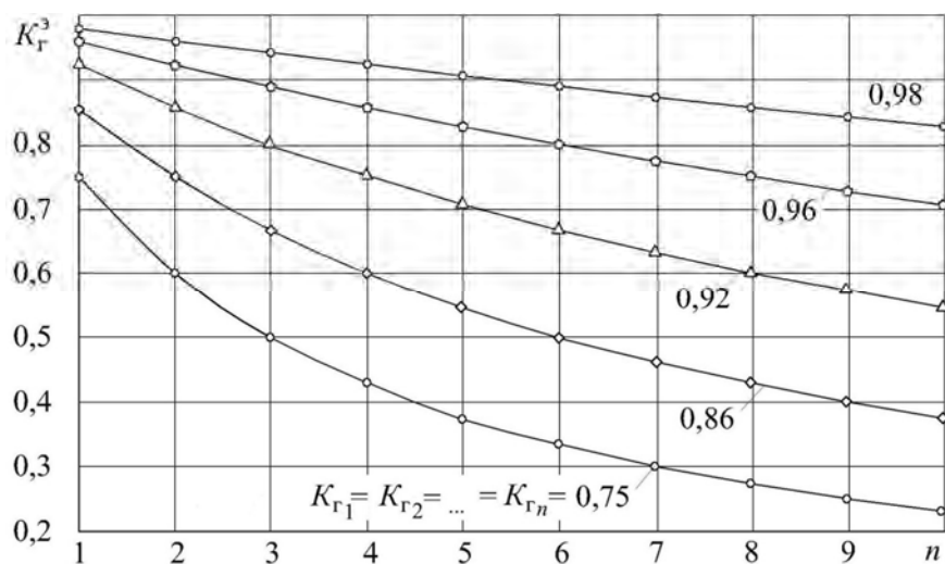
Рисунок 2 – Влияние числа n идентичных ЕТО последовательной компоновки на величину коэффициента K_{Г}^3 готовности ТС при K_{Г_1} = K_{Г_i} = K_{Г_n} , T_{р_1} = T_{р_i} = T_{р_n} и T_{в_1} = T_{в_i} = T_{в_n}
