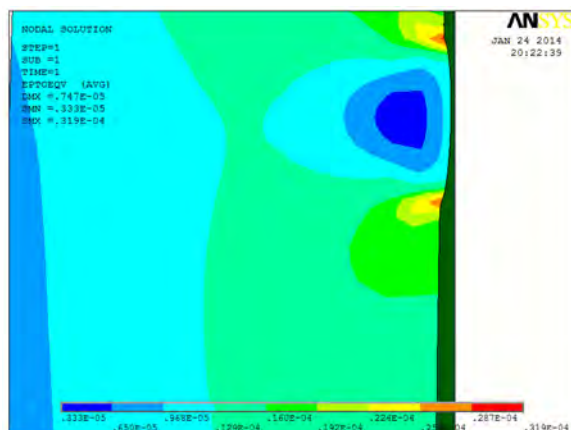
Рисунок 9 – Картина распределения деформаций поверхности вертикального элемента в форме Мизеса в паре металл–полимер в увеличенном виде
