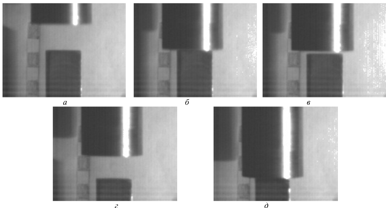
Рисунок 4 – Раскадровка видеосъемки процесса забивания сваи:
