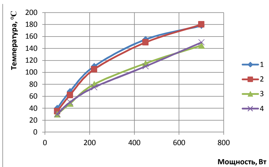
Рисунок 5 – Графики зависимости температуры от мощности тока: 1, 2 – для оправки без втулки; 3, 4 – для втулки
