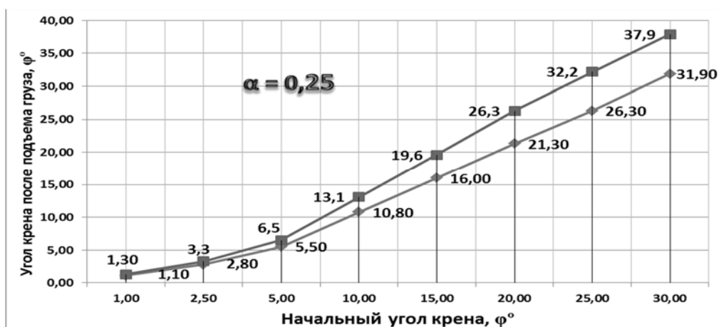
Рисунок 6 – Графики зависимости угла крена судна после подъема груза по расчетному методу и по программе COLOS от начального угла крена судна при \alpha=0,25
