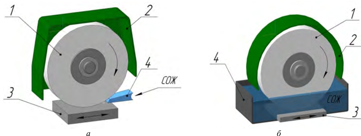
Рисунок 2 – Наиболее значимые способы подачи СОЖ при плоском шлифовании:
