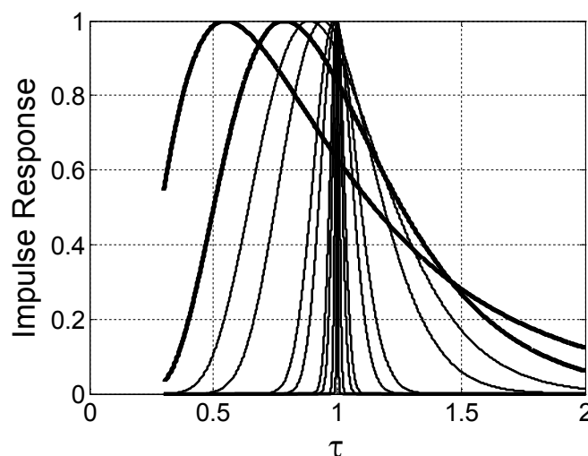
Рисунок 2 – Импульсные характеристики
