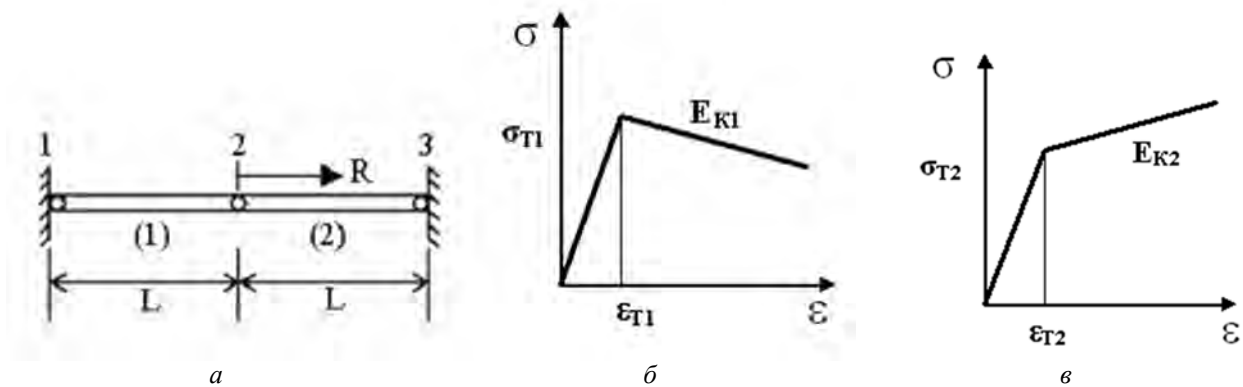
Рисунок 2 – Расчетная схема. Диаграммы деформирования
