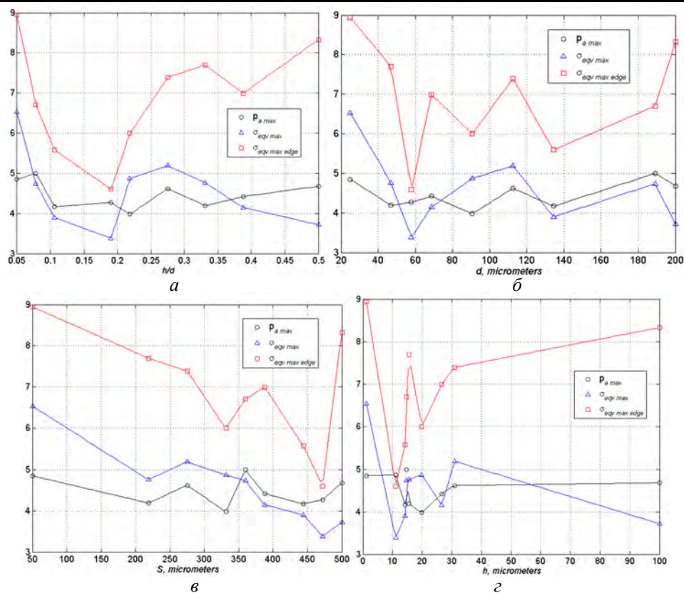
Рисунок 6 – Графики зависимостей критериев p_a \max , \sigma_{eqv \max} и \sigma_{eqv \max edge} в МПа для пары металл–полимер от параметров: а – h/d , б – d в мкм, в – S в мкм, г – h в мкм
