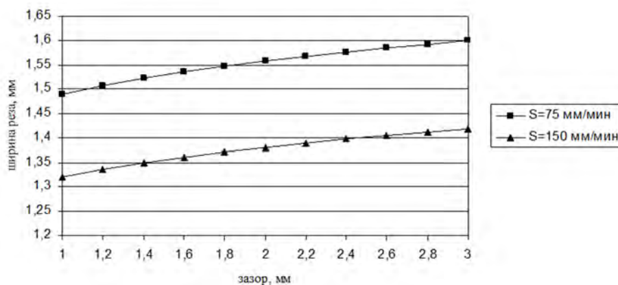
Рисунок 3 – Зависимость ширины реза многослойного материала от межслойного зазора: P = 250 МПа, h = 1 мм
