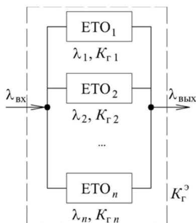
Рисунок 3 – ТС, состоящей из n параллельно соединенных ЕТО:
