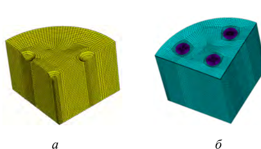
Рисунок 3 – Геометрические модели 1/4 элемента головки без закругления кромок с сеткой конечных элементов: а – с 5 лунками, б – с 12 лунками
