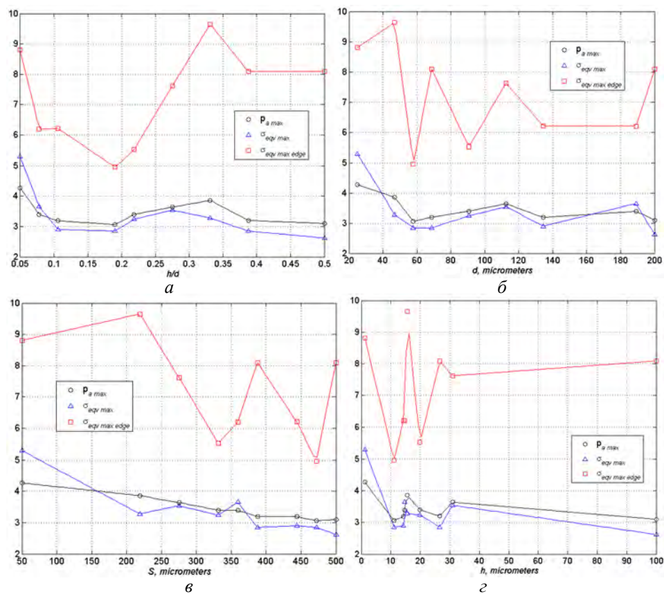
Рисунок 7 – Графики зависимостей критериев p_a \max , \sigma_{eqv \max} и \sigma_{eqv \max edge} в МПа для пары металл–металл от параметров: а – h/d , б – d в мкм, в – S в мкм, г – h в мкм
