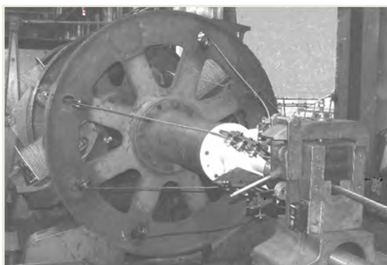
Рисунок 7 – Промышленные испытания шестикасестного преформатора на канатной машине корзиночного типа
