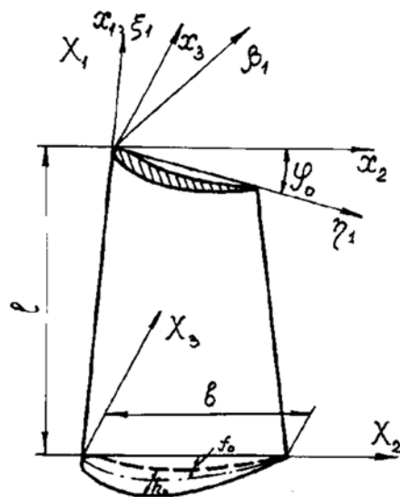
Рисунок 1 – Геометрия и система координат естественно закрученной консольной лопадки
