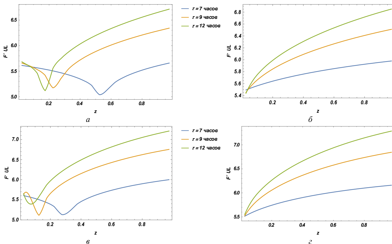
Рисунок 2 – Зависимость F'U_L от координаты z , для различных периодов времени \tau :
