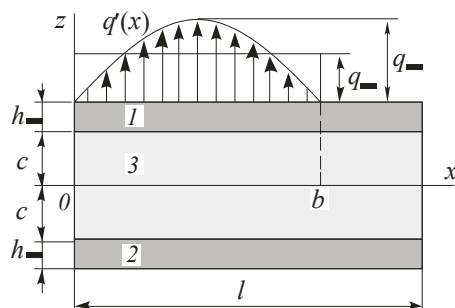
Рисунок 1 – Схема нагружения трехслойного стержня
