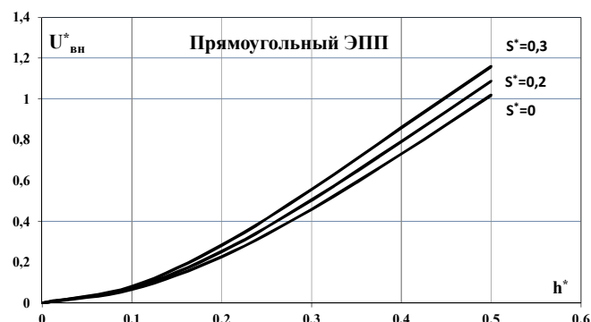
Рисунок 10 – Зависимость U^*_{вн} = U^*_{вн}(h^*, S^*) для прямоугольного ЭПП при R^*_T=2
