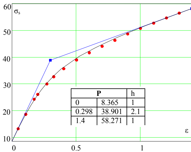
Рисунок 9 – Си-Л90 при растяжении ( t=20^{\circ}\text{C} )
