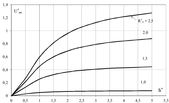
Рисунок 6 – Зависимости U^*_{вн} = U^*_{вн}(h^*, R^*_T) для линейного ЭПП при T \rightarrow \infty
