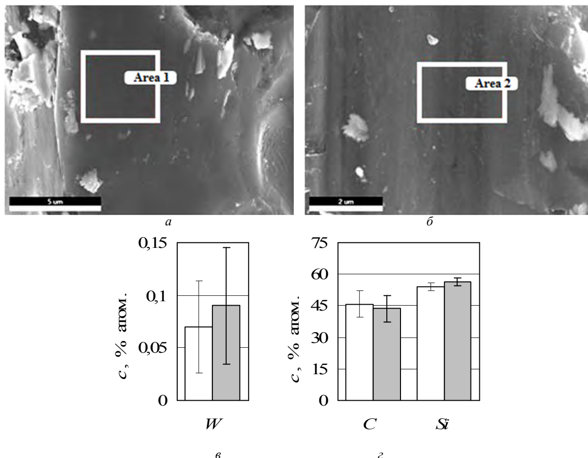
Рисунок 3 – Сканирование относительно чистых участков площадки износа по площади (а, б) и диаграмма концентрации химических элементов (в, з)
