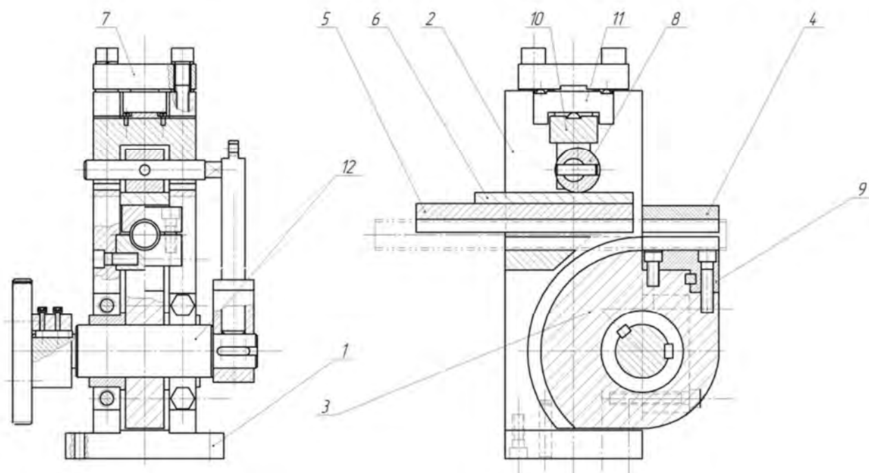
Рисунок 2 – Узел гибки:
