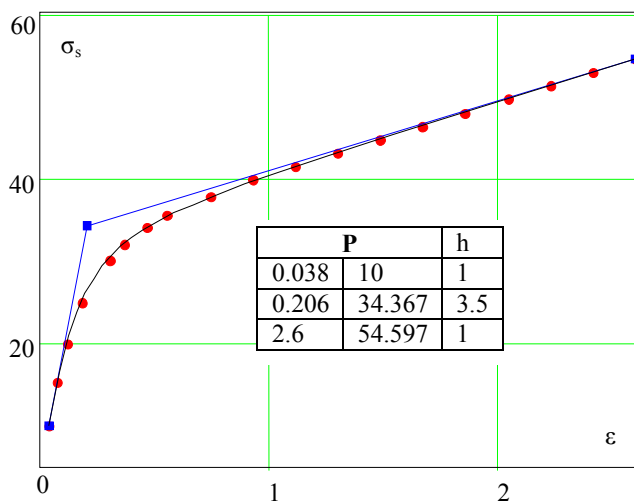
Рисунок 11 – Отожжённая медь М2 при сжатии ( t=20^{\circ}\text{C} )
