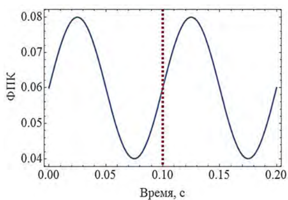
Рисунок 2 – Изменение фактической площади контакта от времени
