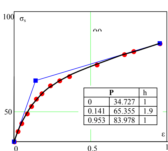
Рисунок 3 – Отожжённая сталь X10Cr13 при сжатии ( t=20^{\circ}\text{C} )
