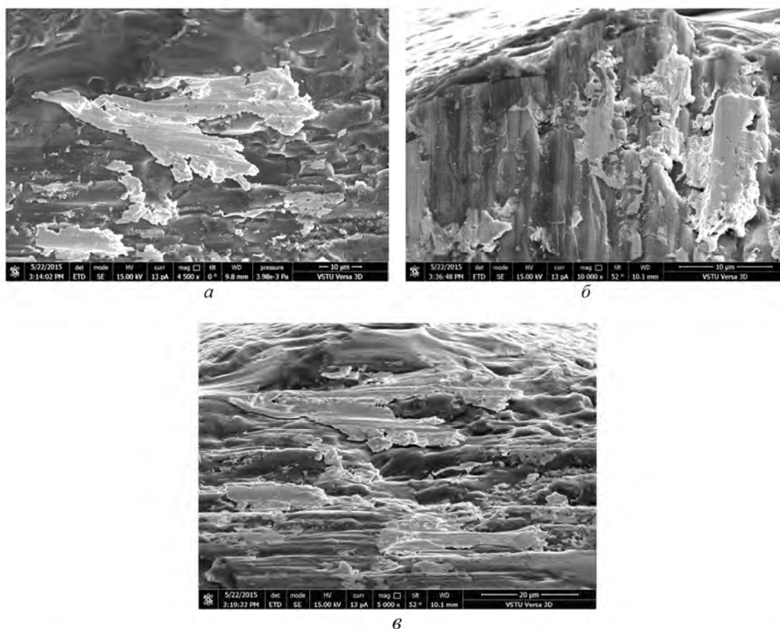
Рисунок 1 – Площадка износа карбида кремния с налипками металла после микроцарапания вольфрама
