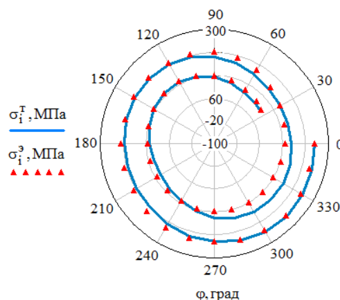
Рисунок 3 – Экспериментальные и теоретические зависимости в координатах \sigma_i = \sigma_i(\varphi)
