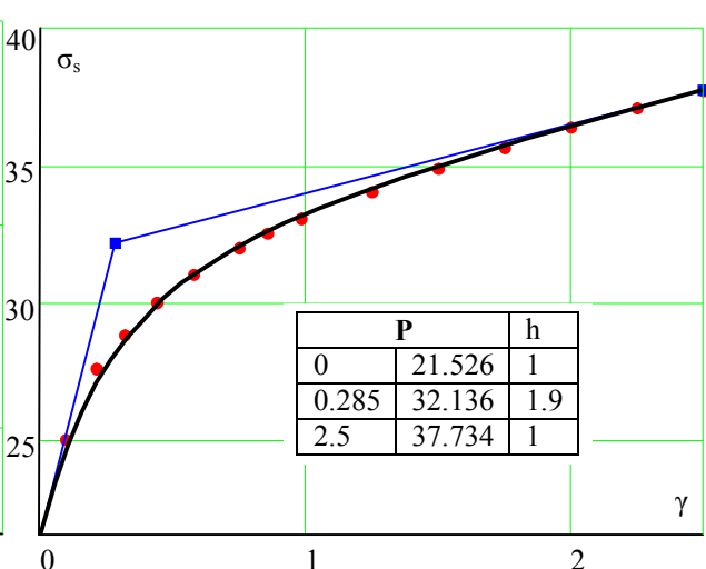
Рисунок 2 – Низкоуглеродистая сталь (C=0,06%) при кручении со скоростью 2,4 \times 10^3 \text{ с}^{-1}
