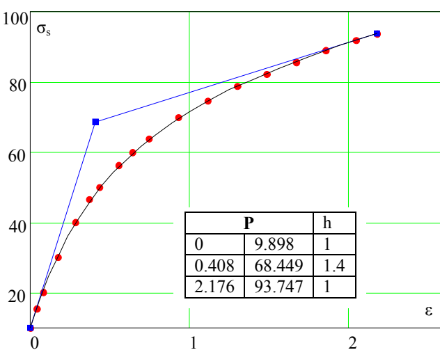
Рисунок 12 – Отожжённая латунь Л63 при сжатии ( t=20^{\circ}\text{C} )
