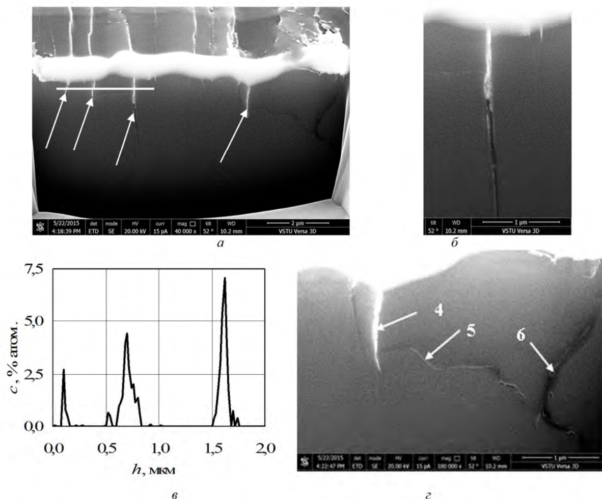
Рисунок 4 – Микросечение поверхности карбида кремния ( а , б , з ) и концентрация кремния по линии сканирования 2 ( в ): а – 40000\times , \alpha=52^\circ ; б – 100000\times , \alpha=52^\circ ; з – 100000\times , \alpha=52^\circ
