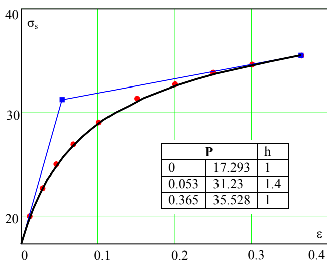
Рисунок 5 – Технически чистая медь, предварительно деформированная холодной осадкой до \epsilon=10\% ( t=20^{\circ}\text{C} )
