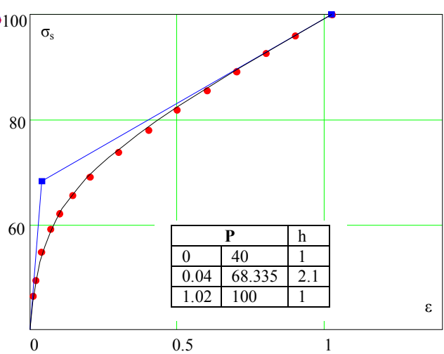
Рисунок 10 – Сталь 30 при растяжении ( t=20^{\circ}\text{C} )
