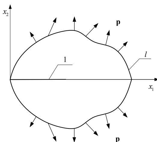
Рисунок 1 – Поперечное сечение тела: l – трещина
