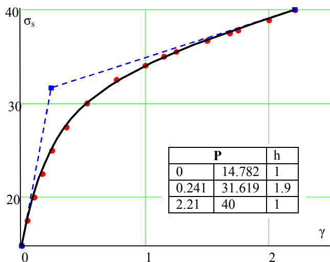
Рисунок 1 – Низкоуглеродистая сталь (C=0,06%) при кручении со скоростью 0,12 \text{ с}^{-1} ( t=78^\circ\text{C} )
