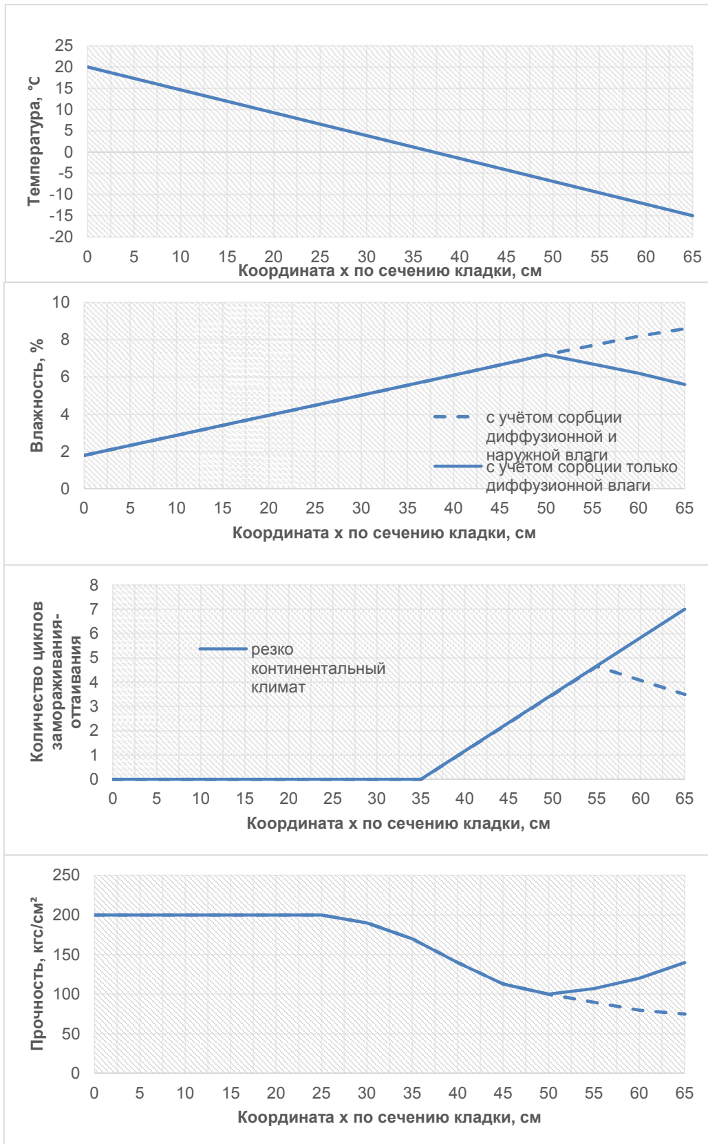
Рисунок 2 – Теоретическое обоснование изменения прочности кладки по сечению наружной стены
