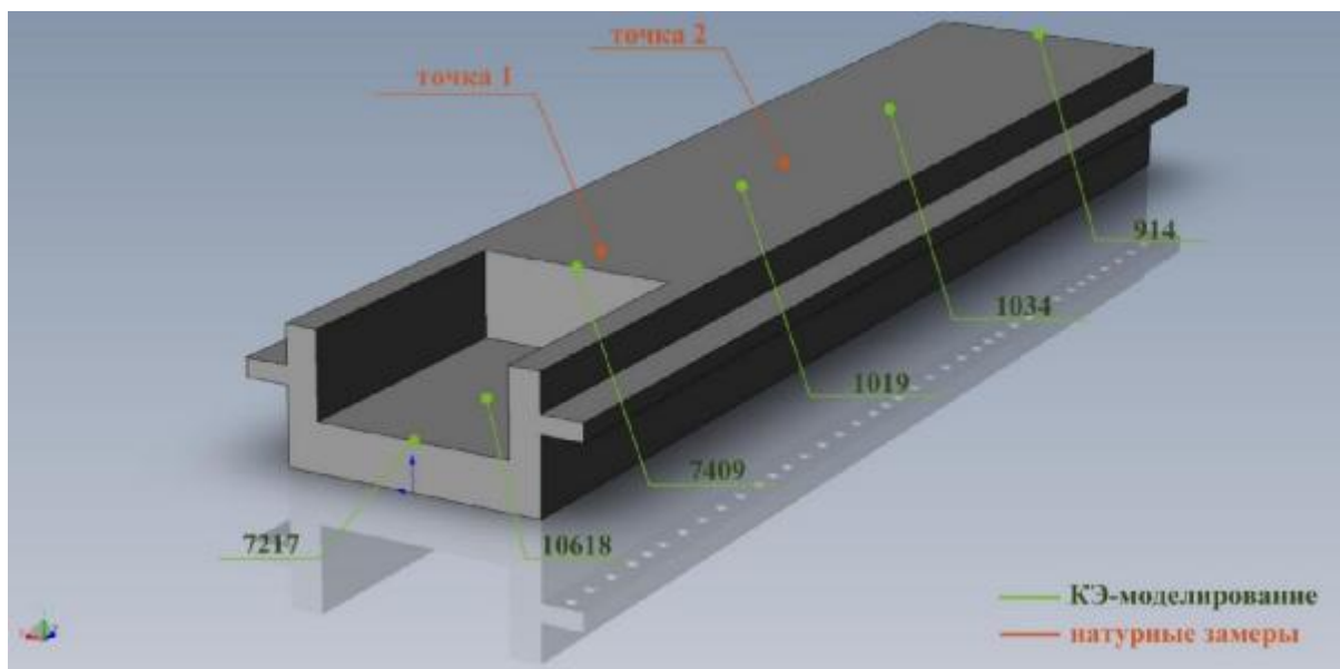
Рисунок 1 – Общий вид фундаментной плиты динамического стенда.
