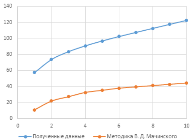
Рисунок 2 – Сравнительный график суммарных тепловых потоков, полученных расчетом температурных полей, и существующей методики для заглубленной стенки
