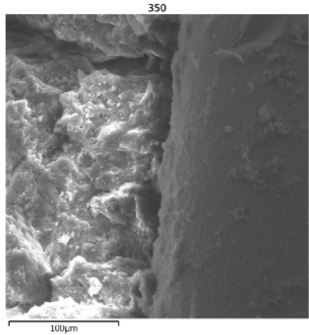
Рисунок 2 – Образец, нагретый до 350 градусов
