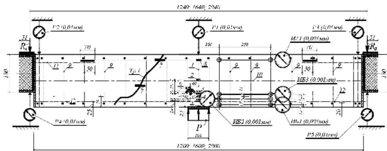
Рисунок 3 – Схема расположения механических приборов и электротензорезисторов, установленных при испытании железобетонных конструкций при действии кручения изгибом :
