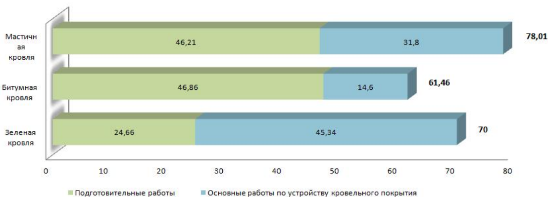
Рисунок 2 – Сравнительная диаграмма трудозатрат при реконструкции кровельных покрытий, чел.-ч./100 кв.м
