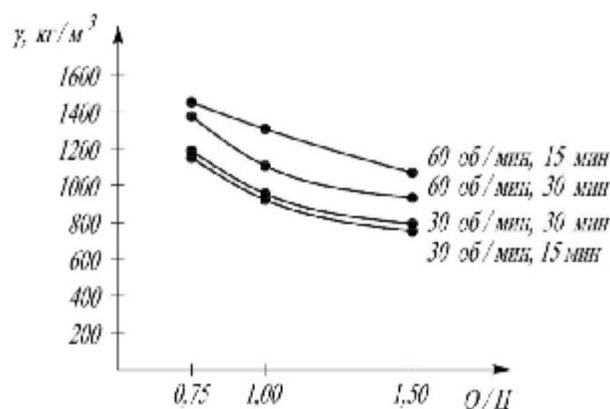
Рисунок 2 – Зависимость плотности \gamma (гамма), кг/м 3 , древесно-цементного материала от технологических параметров смешивания компонентов и состава смеси
