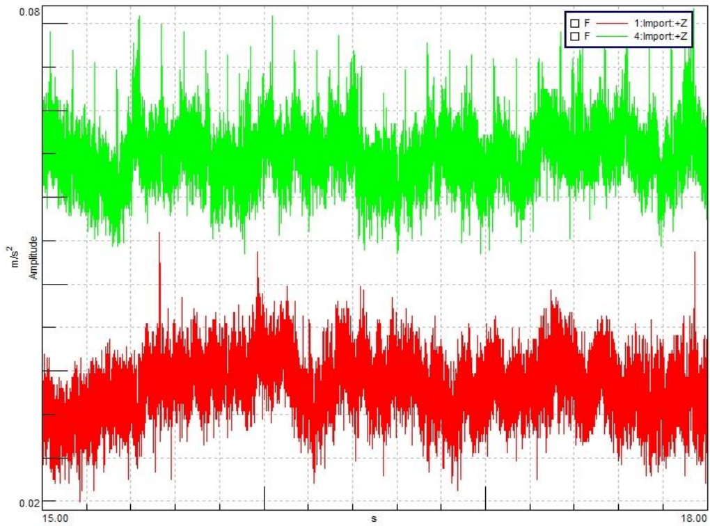
Рисунок 2 – Акселерограмма в точке 1 (зелёная линия) и точке 2 (красная линия) на фундаментной плите
