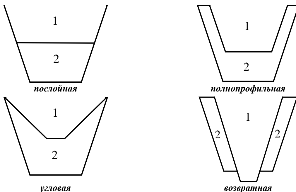
Рисунок 1 – Основные схемы деформирования при режущо-деформирующей обработке резьб в осевом сечении 1- прорезанная канавка; 2- припуск под накатывание
