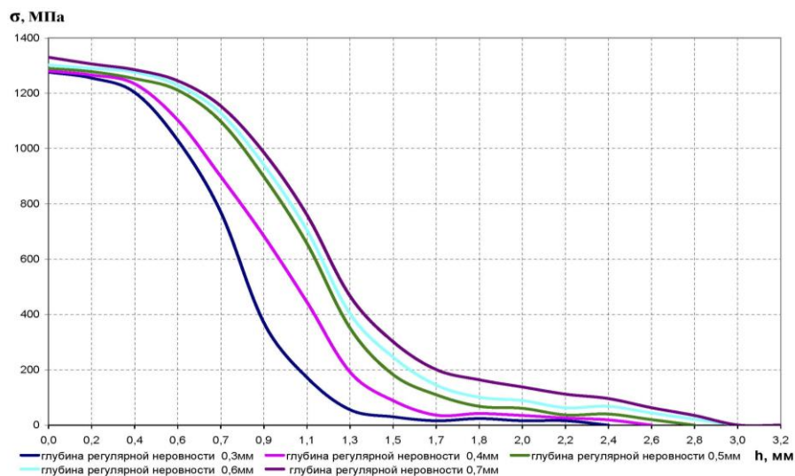
Рисунок 7 – Распределение эквивалентных напряжений \sigma , возникающих по глубине в зависимости от глубины регулярной неровности
