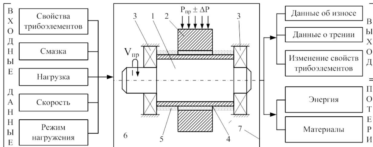
Рисунок 1- Исследуемая модель соединения
