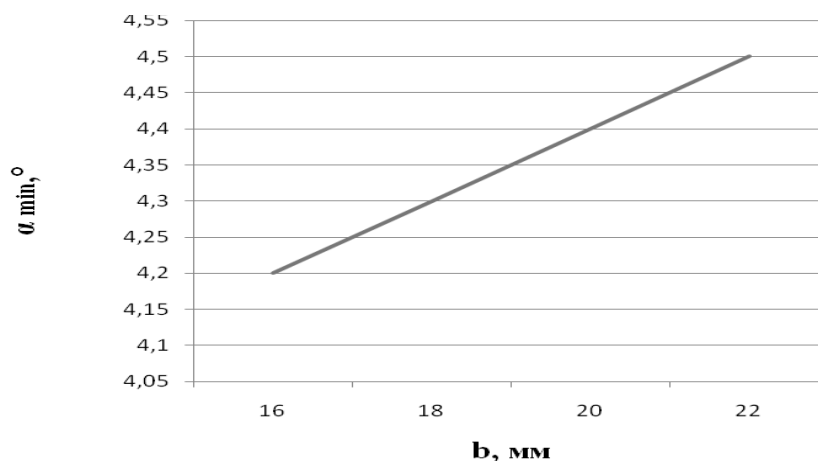
Рисунок 3 – График зависимости минимального значения заднего угла \alpha_{\min} режущего инструмента от ширины b получаемого профиля.
