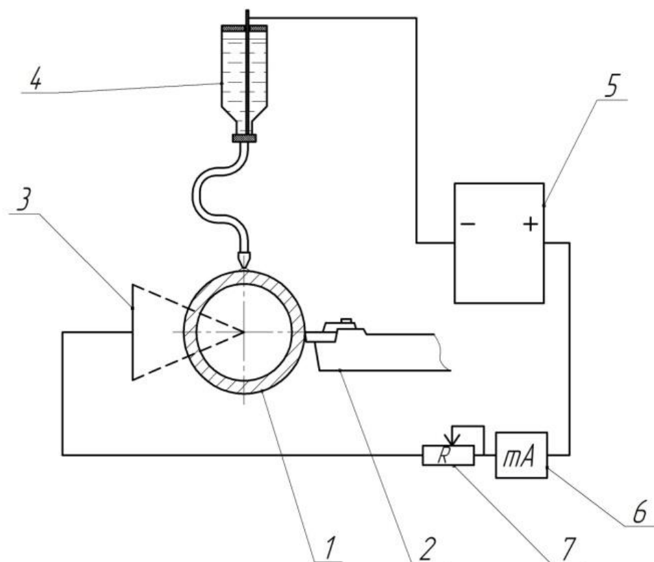
Рисунок 1 - Принципиальная схема установки для комбинированной электрохимической обработки: 1 – заготовка; 2 – режущий инструмент; 3 – динамическое токоёмное устройство; 4 – подача раствора; 5 – источник тока; 6 – микроамперметр; 7 – резистор с регулируемым сопротивлением
