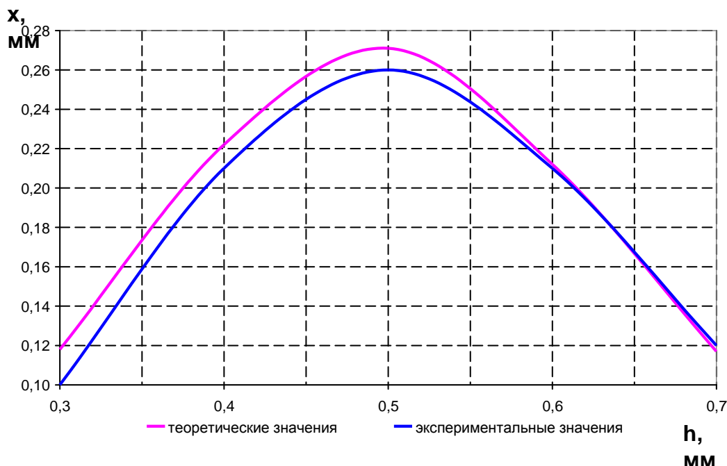
Рисунок 10 – График зависимости подъема металла x от глубины регулярной неровности h
