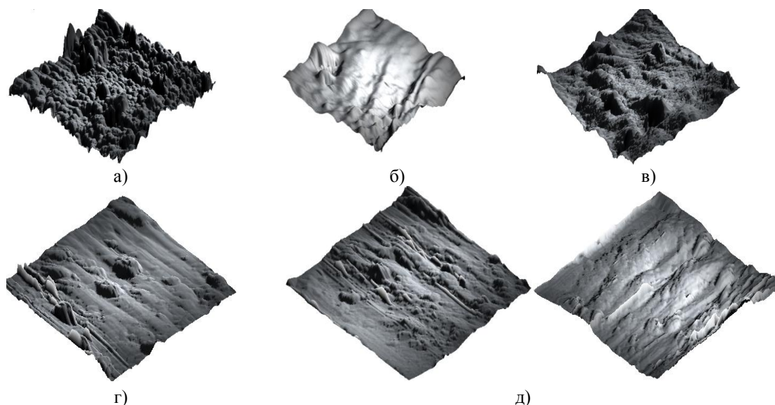
Рисунок 1 - Морфология нитрида титана, модифицированного фторсодержащим олигомером Ф-АК-1 а) нитрид титана; б) нитрид титана+Ф-АК1; в) нитрид титана+Ф-АК1 + термообработка при T=373K ; г) нитрид титана+Ф-АК1 + термообработка при T=473K ; д) нитрид титана+Ф-АК1+ термообработка при T=523K . Площадь сканирования 25x25 мкм.
