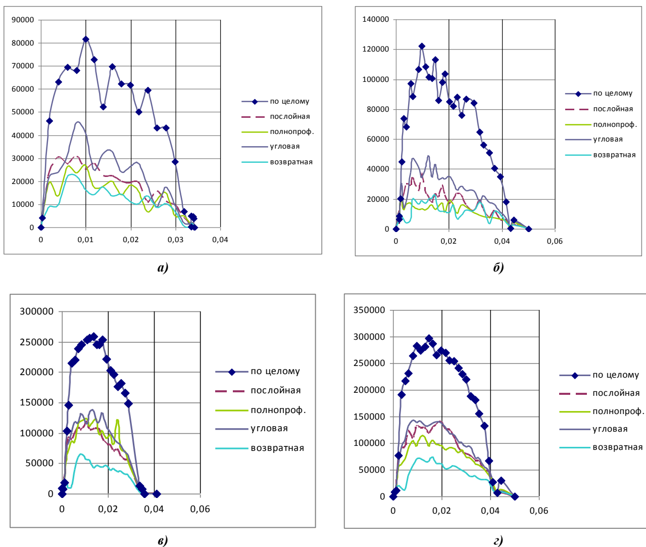
Рисунок 3 – Графики зависимости сил деформирования от времени накатывания при различных схемах деформирования
