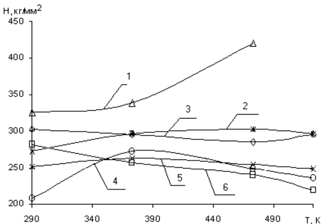
Рисунок 2 - Зависимость микротвердости от температуры термообработки подложек 1-нитрид титана + фторопласт после коррозионных испытаний; 2-нитрид титана + Ф-АК1; 3-нитрид титана; 4-нитрид титана+Ф-АК2; нитрид титана+Ф-14; нитрид титана + фторопласт
