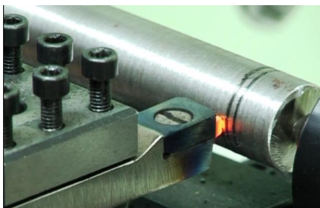
Рисунок 4 - Высадка изношенной поверхности
