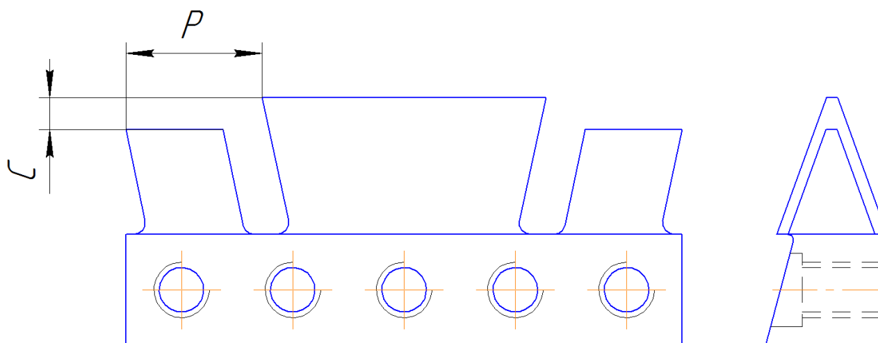
Рисунок 1 – Конструкция инструмента
