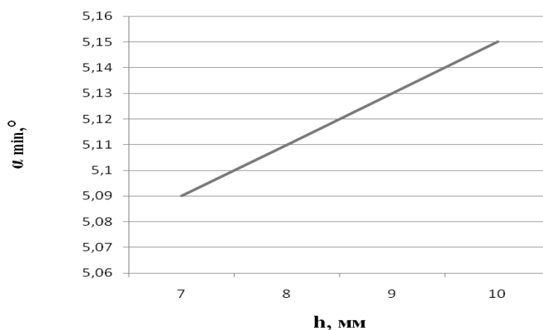
Рисунок 4 – График зависимости минимального значения заднего угла \alpha_{\min} режущего инструмента от высоты h получаемого профиля.
