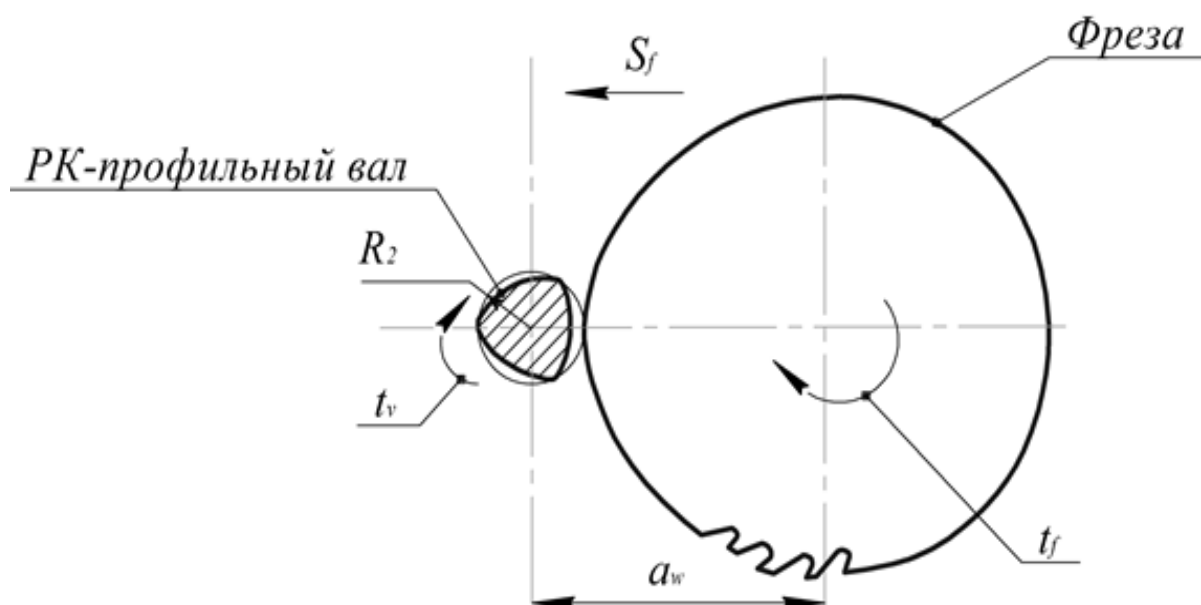
Рисунок 1 - Схема обработки валов с равноосным контуром дисковой фрезой с переменным радиусом
