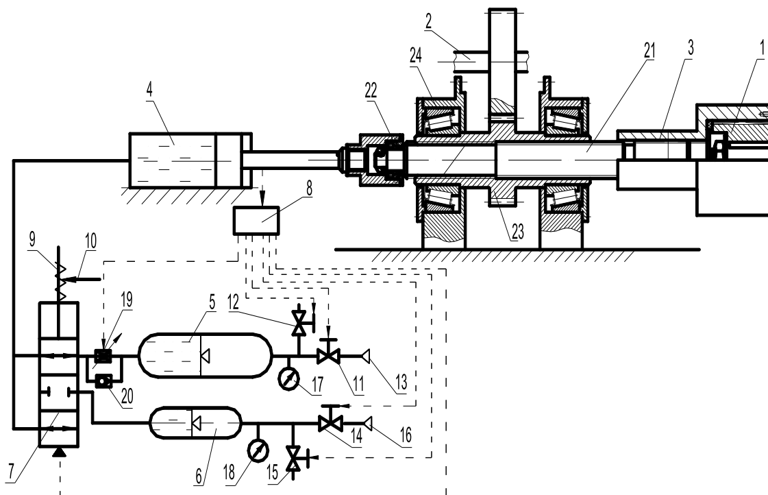
Рисунок 1 – Гидромеханическая муфта с дифференциальным передаточным механизмом винт-гайка 1, 2 – полумуфты; 3 – шлицевая втулка; 4 – гидроцилиндр; 5 – гидропневмодемпфер; 6 – гидропневмоаккумулятор; 7 – гидрораспределитель; 8 – система управления; 9 – упругий элемент; 10 – фиксатор; 11, 12, 14, 15 – вентили; 13 – источник высокого давления газа; 16 – источник низкого давления газа; 17, 18 – датчики давления; 19 – гидродроссель; 20 – обратный клапан; 21 – винт; 22 – упорный подшипник; 23 – гайка; 24 – подшипник
