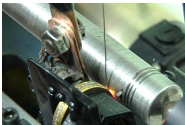
Рисунок 5 – Приваривание дополнительного материала
