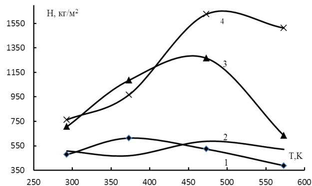
Рисунок 7 - Значения микротвердости (кг/м²) алмазоподобных покрытий 1,3-исходные; 2,4-модифицированные фторсодержащим олигомером Ф1; 1,2- образец №1; 3,4-образец №2
