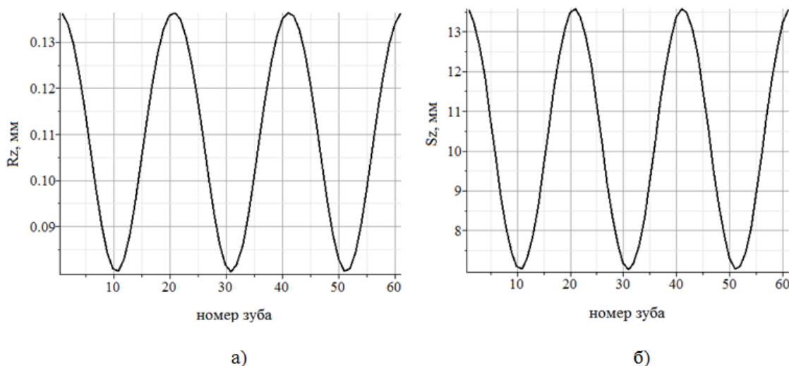
Рисунок 3 - График изменения параметров остаточного гребешка
