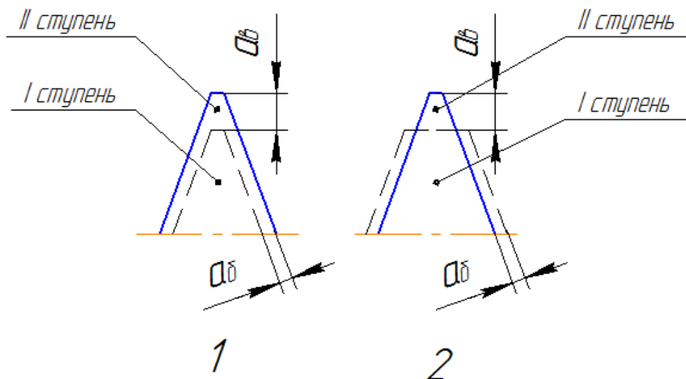
Рисунок 2 – Взаимное расположение режущих лезвий
