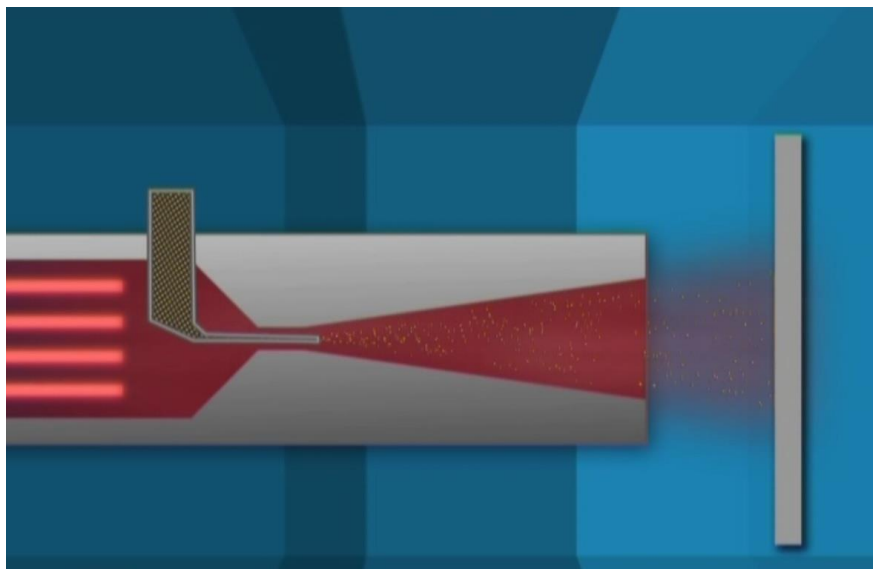
Рисунок 6 - Газодинамический метод нанесения покрытий
