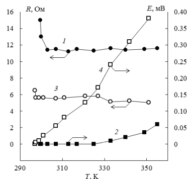
Рисунок 3 – Зависимость от температуры слоя шарообразных частиц меди электрического сопротивления слоя (1), (3) и термоэдс в этом слое (2), (4) до (1), (2) и после (3), (4) воздействия на этот слой атомарным водородом в течение 5 ч.
