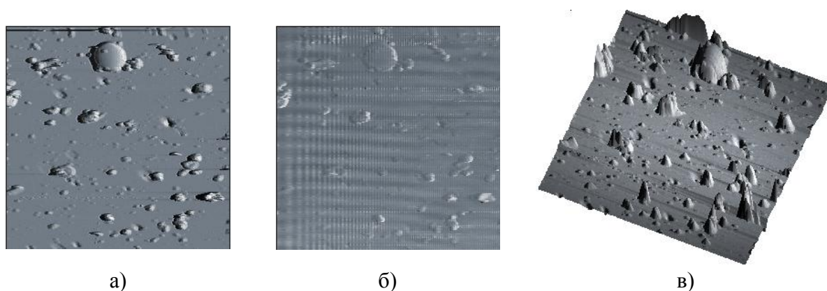
Рисунок 5 - Алмазоподобное покрытие на стальной подложке (образец №2) а) топография, б) фазовый контраст, в) 3D-изображение, площадь сканирования 25х25 мкм
