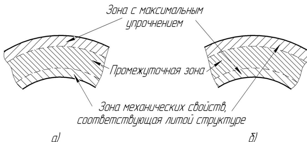
Рисунок 2 - Принципиальная схема по распределению механических свойств втулок, обработанных по способам [5, 6]
