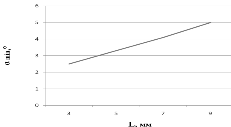
Рисунок 2 – График зависимости минимального значения заднего угла \alpha_{\min} режущего инструмента от ширины режущей кромки L .
