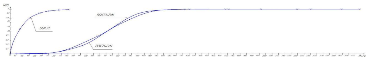
Рисунок 2 - Зависимость вероятностей отказа от времени
