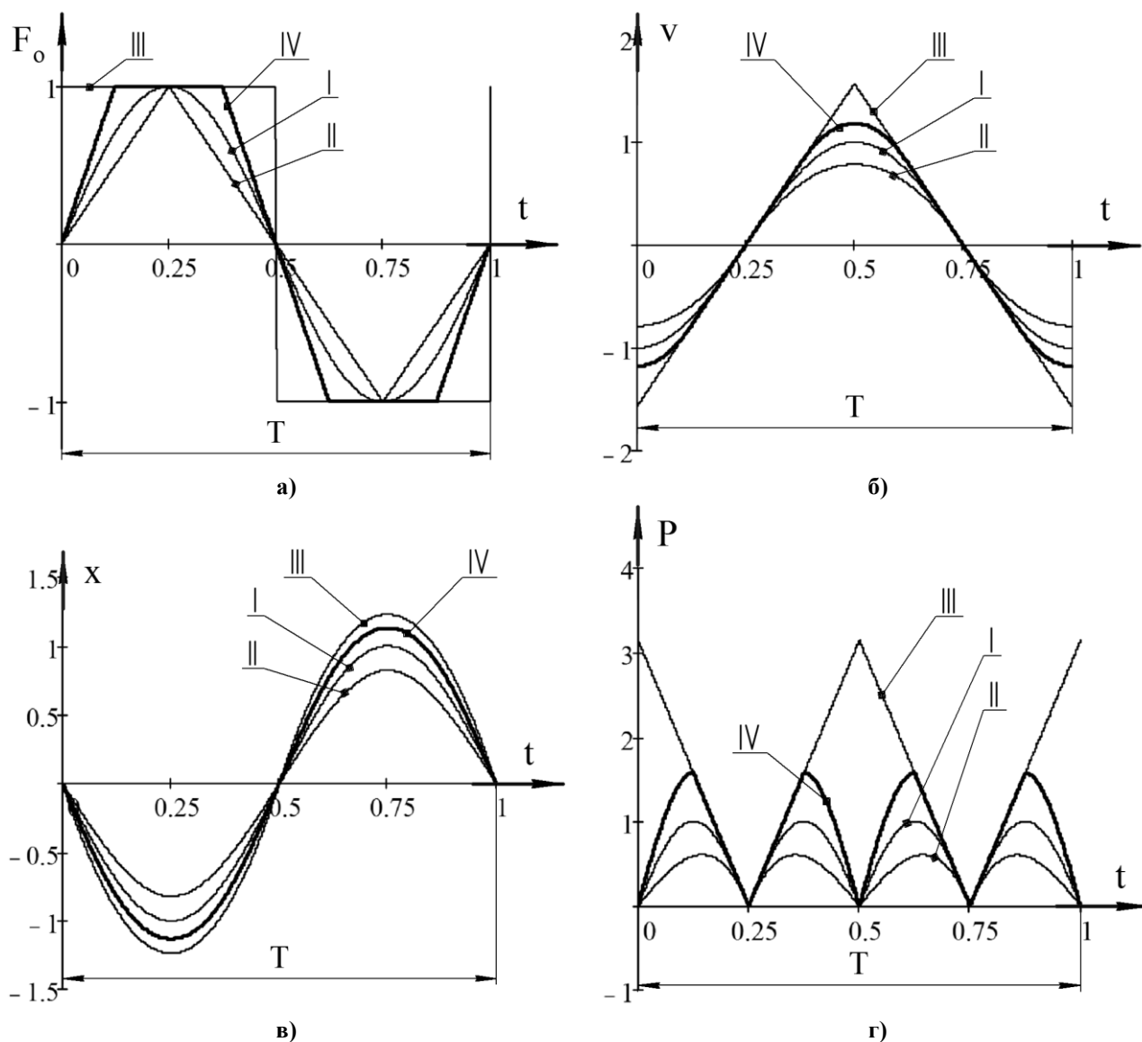
Рисунок 2 – Диаграммы изменения возмущающей силы (а), скорости (б), координаты (в) и мощности (г) при поперечных колебаниях колебательной системы по законам I – синусоидальному; II – пилообразному; III – прямоугольному; IV - трапецеидальному
