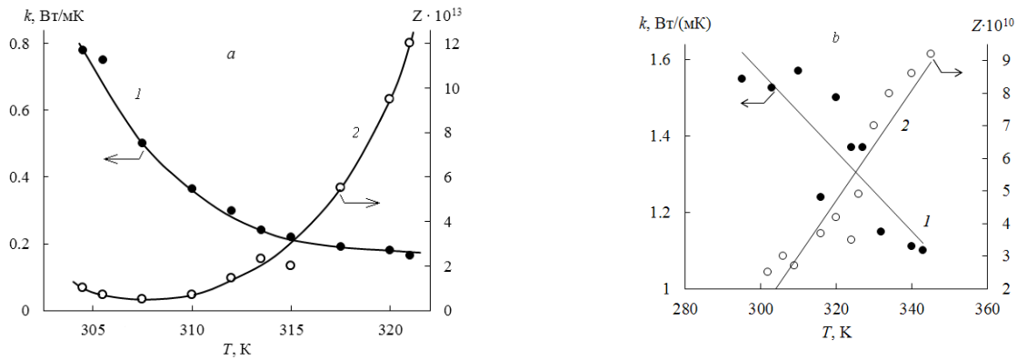
Рисунок 4 – Зависимость коэффициента теплопроводности (1) и термоэлектрической эффективности (2) слоя шарообразных частиц меди от температуры до (а) и после (б) воздействия на этот слой атомами водорода в течение 5ч.
