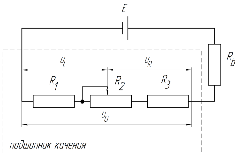
Рисунок 4 – Электрическая схема подключения узла трения экспериментальной установки
