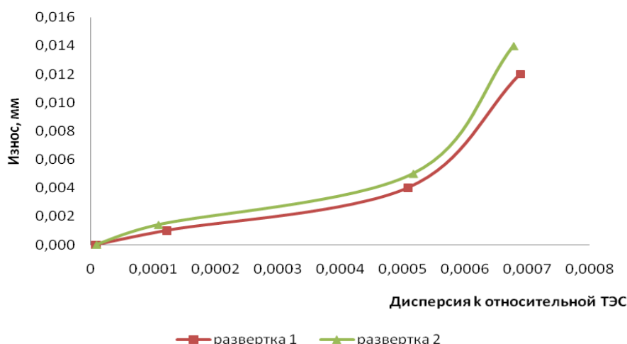
Рисунок 2 - Зависимость изменения линейного износа режущих кромок развертки от дисперсии к относительной ТЭС
