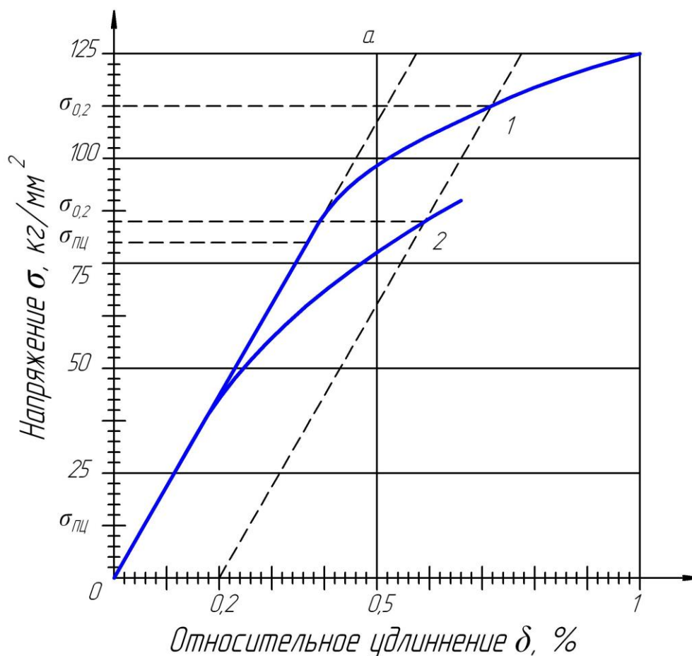
Рисунок 2 – Изменение величины предела пропорциональности \sigma_{0,2} при прямой и реверсивной деформации 1 – материал не подвергавшийся деформации, 2 – после деформирования его нагрузкой обратного знака.
