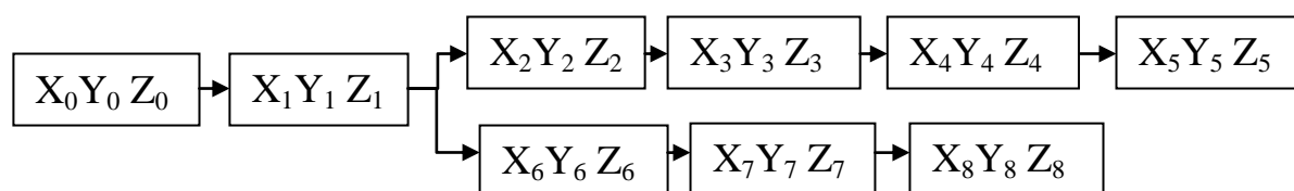
Рисунок 3 - Структура формообразующей системы агрегатного станка
