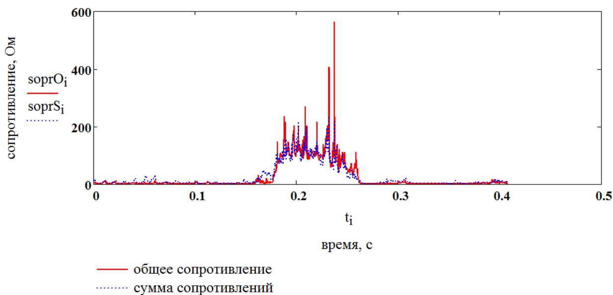
Рисунок 6 – Иллюстрация близости формы временных диаграмм суммарного и полного электрического сопротивления
