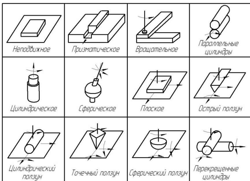
Рисунок 1 – Классификация соединений
