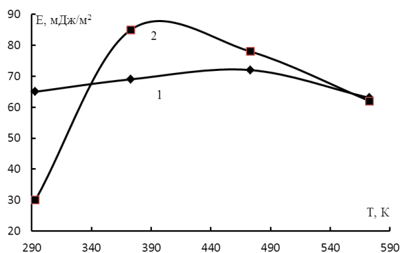
Рисунок 6 - Значения поверхностной энергии для алмазоподобного покрытия в зависимости от различных режимов термической обработки 1 – исходная, 2 – обработанные ФСО Ф1
