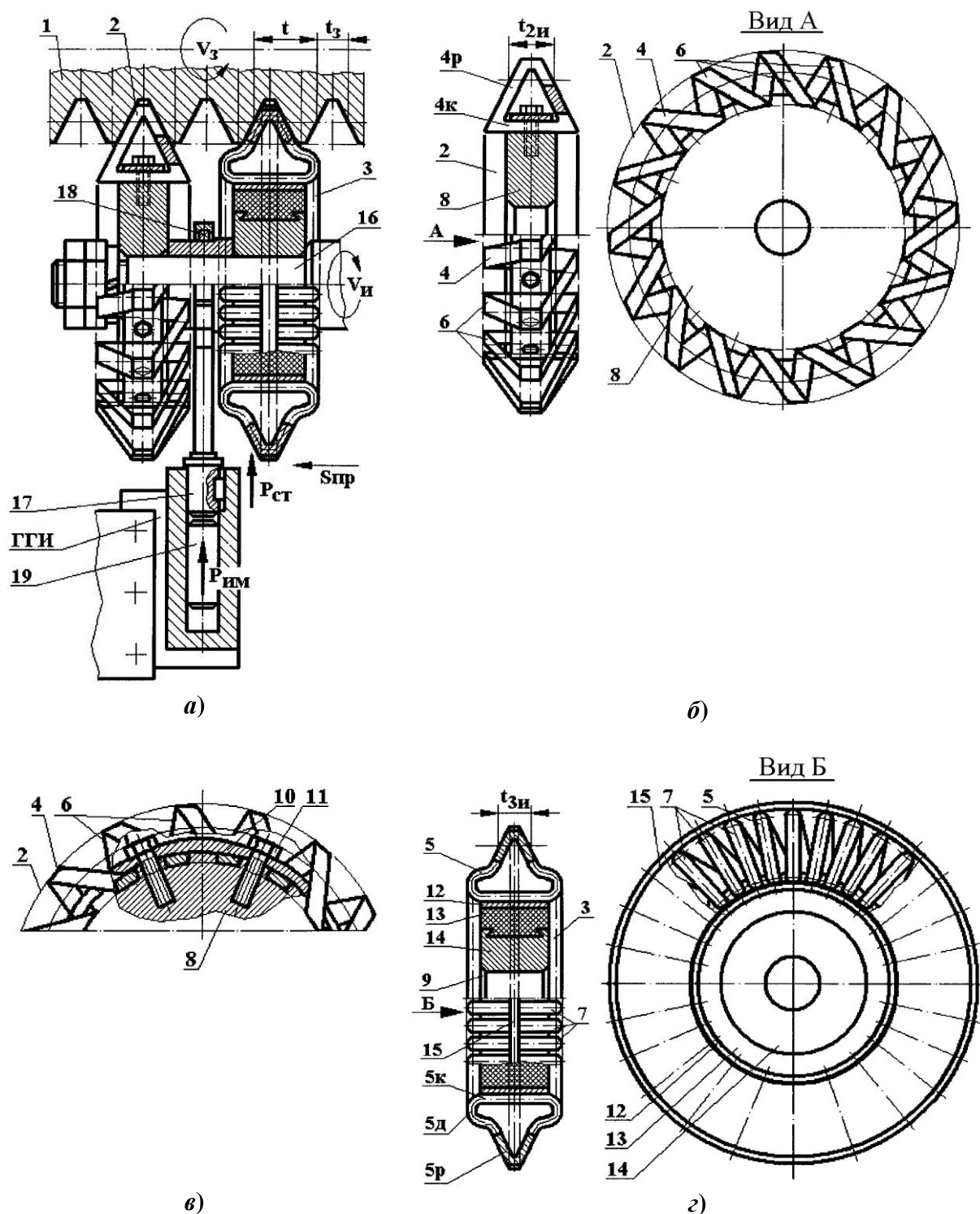
Рисунок 1 – Устройство для упрочнения резьбы:
