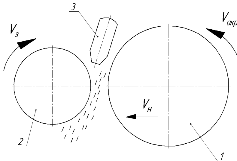
Рисунок 2 — Схема электроэрозионного шлифования 1 — электрод — инструмент; 2 — заготовка; 3 — насадка
