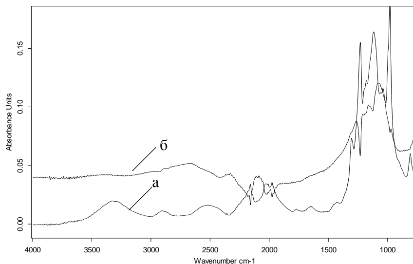
Рисунок 3 – ИК-спектр алмазоподобного покрытия (образец №1) а – с пленкой ФСО Ф1, б – исходное покрытие
