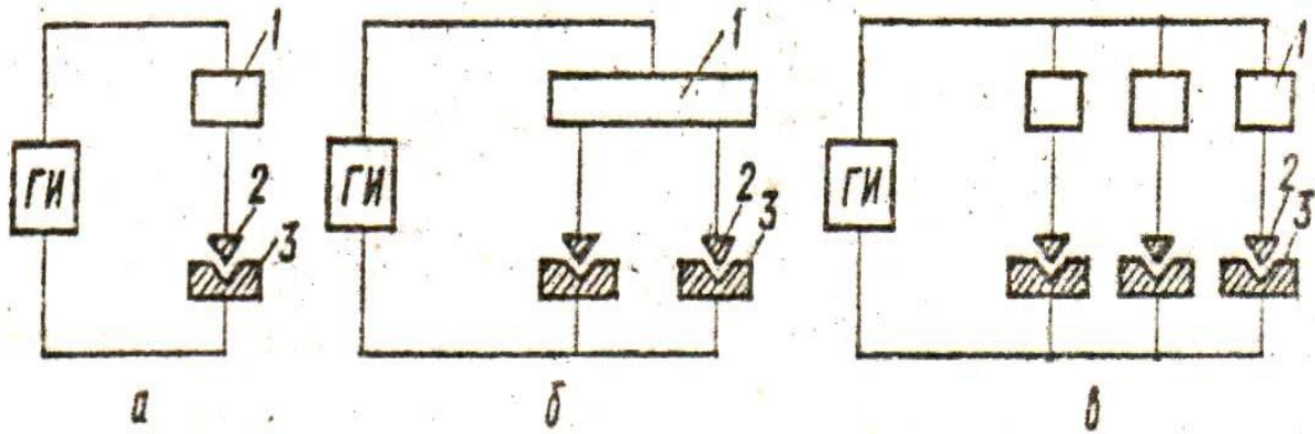
Рисунок 1 - Изготовление полостей на крупногабаритных штампах и пресс-формах
