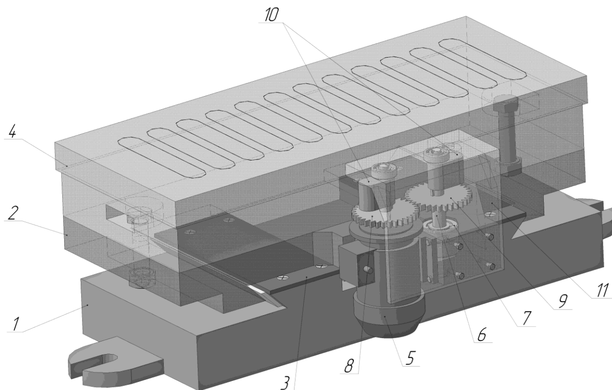
Рисунок 1 – Инерционная установка для виброшлифования:
