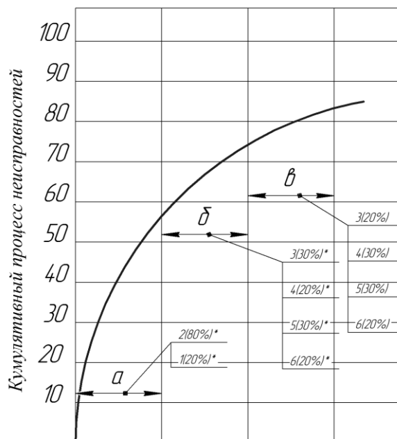
Основные виды неисправностей (а, б, в, - см. рисунок 1) из-за проявления деструктивных факторов (1, 2, 3, 4, 5, 6 - см. рисунок 1) на стадиях испытания, доводки и эксплуатации
