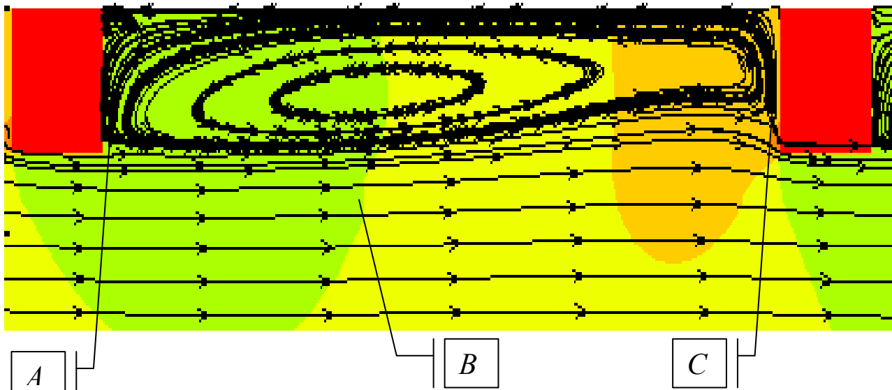
Рисунок 2 - Линии тока для случая ( Re=10^4 ; d/D=0.94 ; t/D=0.25 , воздух)
