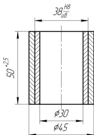
Рисунок 3 - Эскиз запрессованной втулки
