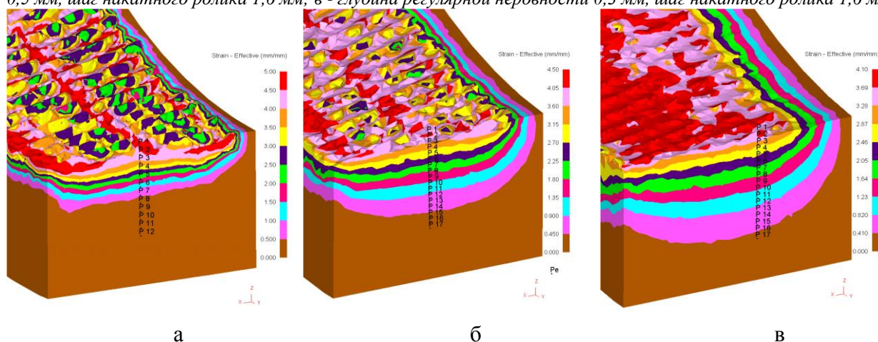
Рисунок 6 – Поля эквивалентных деформаций \varepsilon , возникающих по глубине
