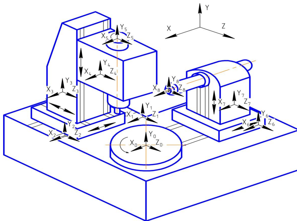
Рисунок 1 - Формообразующая система агрегатного станка.
