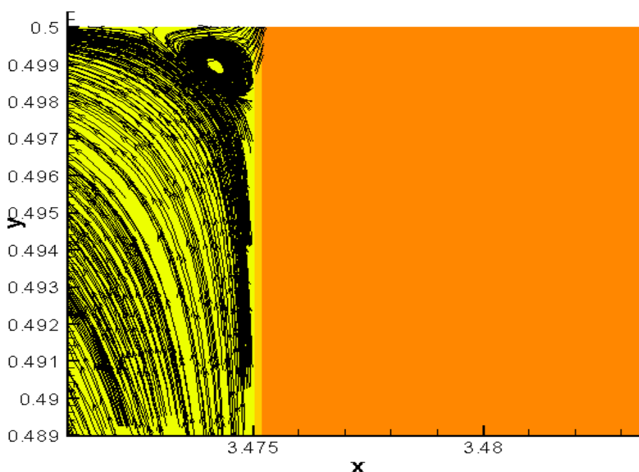
Рисунок 4 - Структура потока при ( Re=10^4 ; d/D=0.90 ; t/D=1.00 , воздух)
