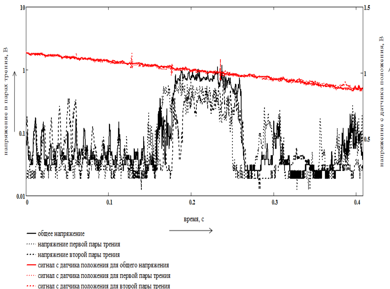
Рисунок 5 – Временные диаграммы изменения измеряемых напряжений
