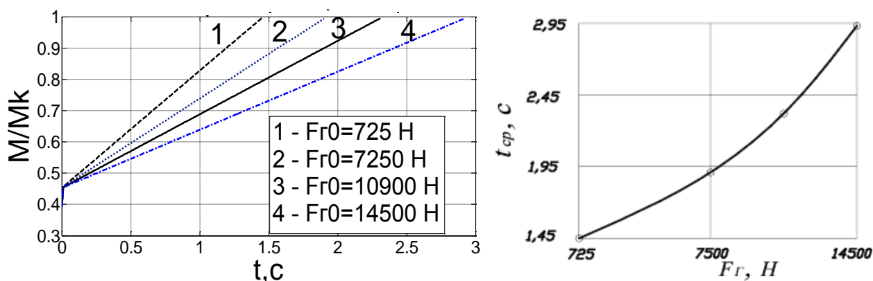
Рисунок 2 – Влияние начального усилия на штоке гидроцилиндра на момент и время срабатывания муфты
