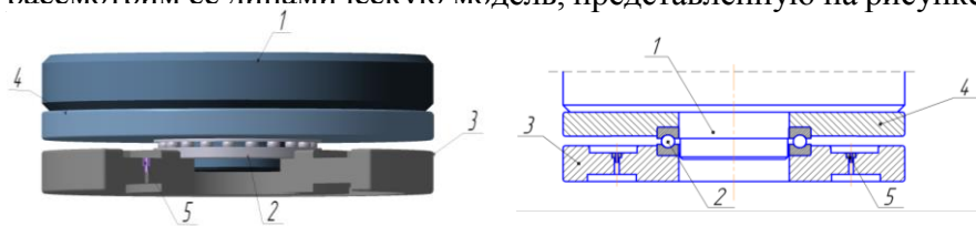
Рисунок 1 – 3D-модель и схема упорной совмещенной опоры 1-Вал; 2-Подшипник качения; 3-Пята подшипника скольжения; 4-Подпятник подшипника скольжения; 5-Система подачи смазочного материала
