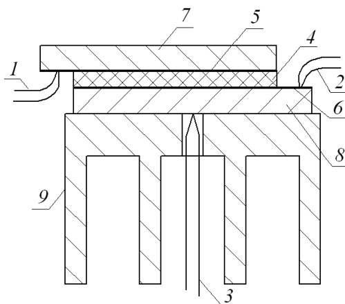
Рисунок 1 – Схема устройства для измерений коэффициента теплопроводности и термоэлектрической эффективности материала, состоящего из шарообразных наночастиц 1,2,3 – термопары для измерений температур T_1 , T_2 и T_3 соответственно; 4 – слой наночастиц; 5 и 6 – электроды (алюминиевые пленки) на поверхности пластинок кремния 7 и 8; 9 – радиатор. Электрические контакты к электродам 5 и 6 на схеме не показаны.
