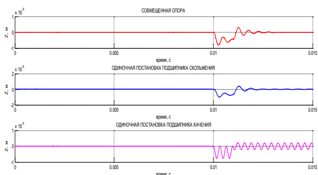
Рисунок 3 – Сравнительный анализ разверток осевых колебаний совмещенной опоры
