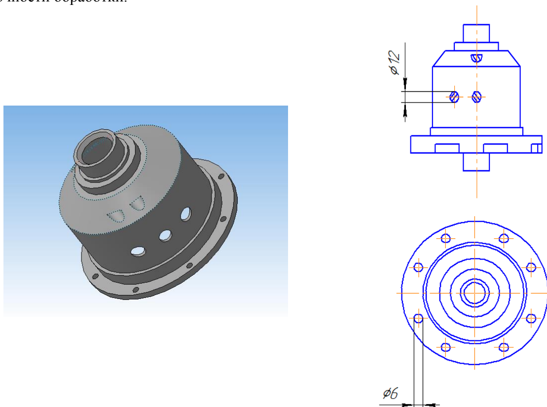
Рисунок 2 - Обрабатываемая деталь
