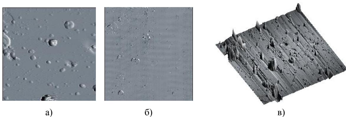
Рисунок 4 - Алмазоподобное покрытие на стальной подложке (образец №1) а) топография, б) фазовый контраст, в) 3D-изображение, площадь сканирования 10х10 мкм
