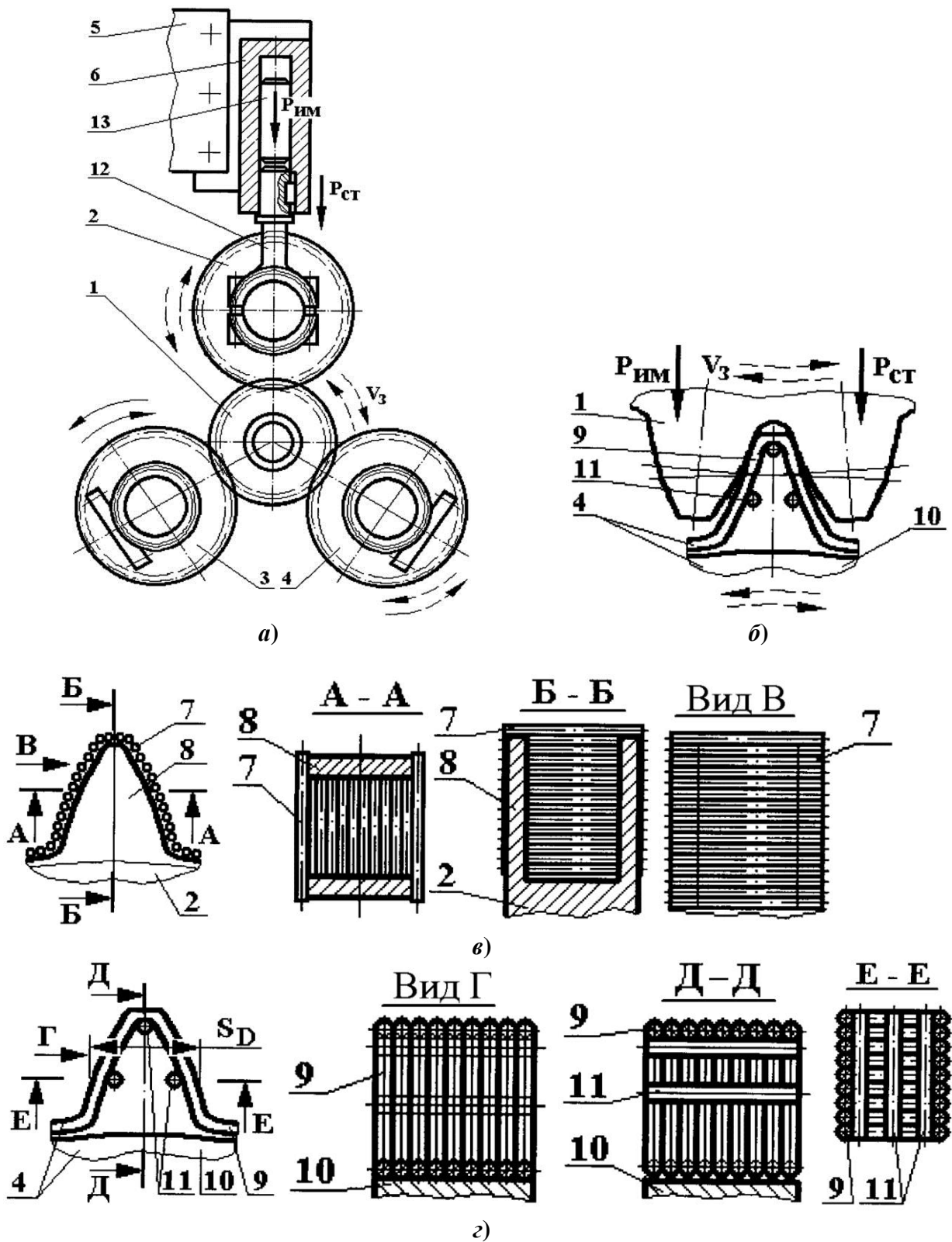
Рисунок 2 – Устройство для статико-импульсного обкатывания зубчатых колес:
