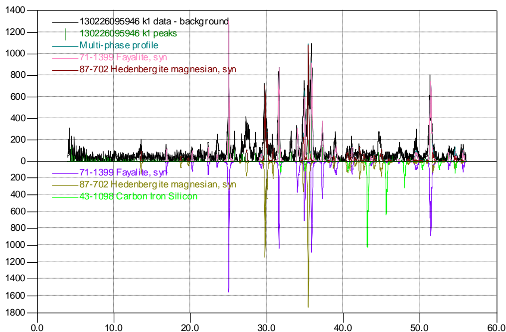
Рисунок 2- Рентгенофлуоресцентный анализ образцов модифицированного материала
