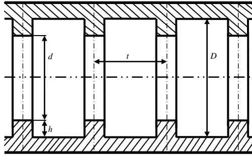
Рисунок 1 - Основные геометрические параметры турбулизаторов
