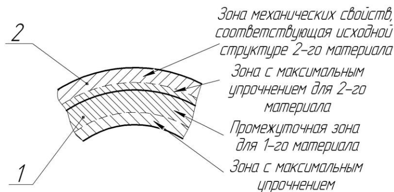
Рисунок 4 - Принципиальное распределение механических свойств биметаллических втулок, обработанных по способу [6].
