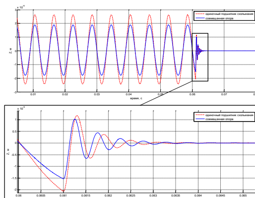
Рисунок 4 – Сравнительный анализ разверток осевых колебаний совмещенной опоры в случае возбуждения гармоническими колебаниями
