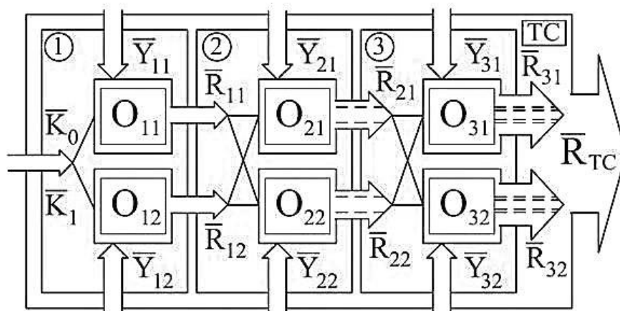
Рисунок 2 - Структура комбинированной антифрикционной обработки
