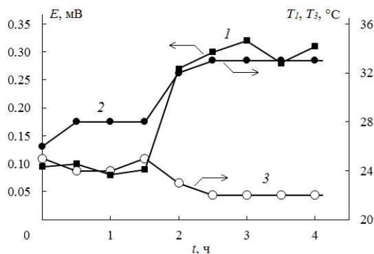
Рисунок 2 – Зависимость от времени выдержки в среде атомарного водорода подложки с нанесенным слоем шарообразных частиц меди термоэдс в не нагреваемой светом части слоя частиц меди (1), температуры поверхности, не нагреваемой светом части этого слоя (2), и температуры нижней поверхности подложки (3)
