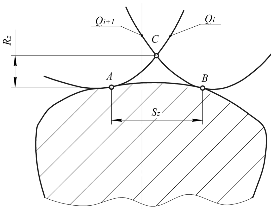
Рисунок 2 - Схема расчета параметров остаточных слоев
