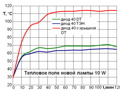
Рисунок 5 - Результаты измерения температуры внутри светодиодной лампы
