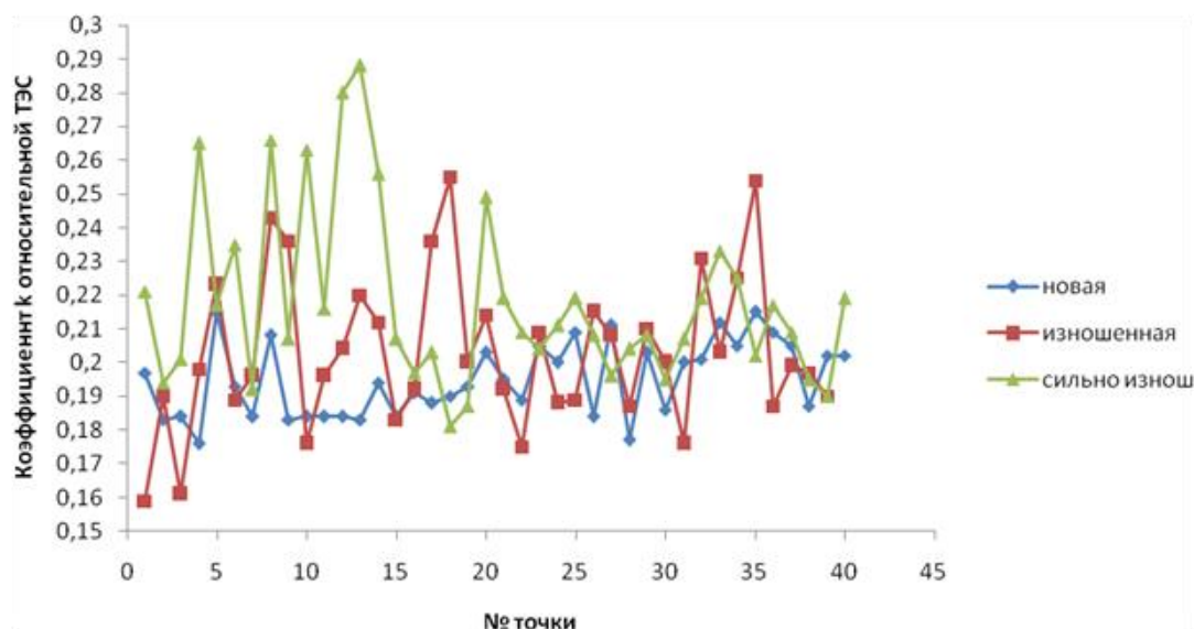
Рисунок 1 - График изменения коэффициента k относительной ТЭС для различных точек поверхностей режущих кромок разверток с различной степенью износа
