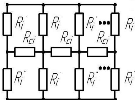
Рисунок 1 - Упрощенная параллельно-последовательная электрическая эквивалентная схема подшипника R_i' - сопротивления трибосопряжения в зонах контакта тел качения и дорожки внутреннего кольца, R_i'' - сопротивление трибосопряжения в зонах контакта тела качения и дорожки внешнего кольца, R_{ci} - дополнительное сопротивление трибосопряжения в зонах контакта тел качения и сепаратора
