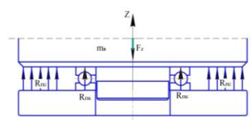
Рисунок 2 – Динамическая модель упорного совмещенного подшипникового узла гидростатического типа
