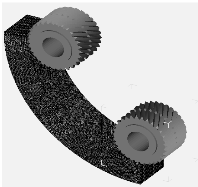
Рисунок 3 – Заготовка со сформированной конечно-элементной сеткой (500000 элементов)
