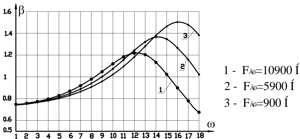
Рисунок 3 – Коэффициент динамичности муфты при начальных давлениях в гидродемпфере
