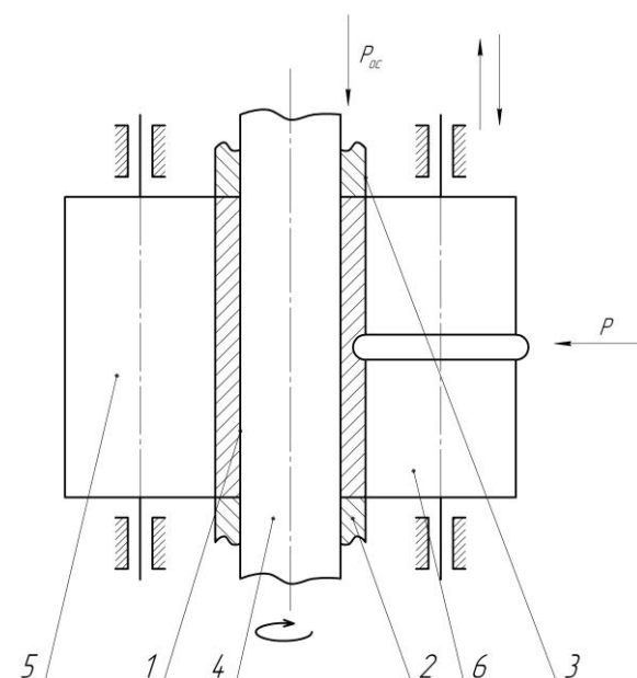
Рисунок 1 - Схема способа получения полых осесимметричных изделий с градиентным от наружной поверхности субмикро- или наноструктурным состоянием материала:
