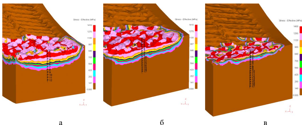
Рисунок 5 - Поля эквивалентных напряжений \sigma , возникающих по глубине
