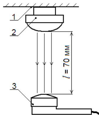
Рисунок 2 - Схема измерения освещённости 1 – потолок, 2 – лампа, 3 – датчик люксметра
