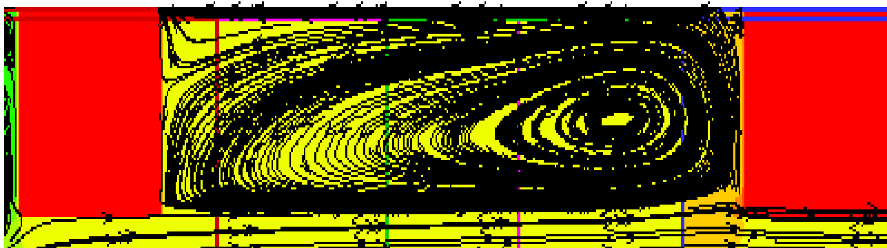
Рисунок 3 - Линии тока для случая ( Re=10^4 ; d/D=0.94 ; t/D=0.5 , воздух)
