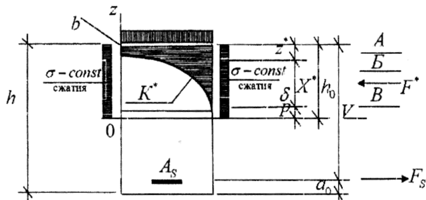
Рисунок 1 – Схема распределения коррозионных повреждений в сечении изгибаемой балки (A – зона полного повреждения; B – зона частичного повреждения; B – зона неповрежденной части сечения)
