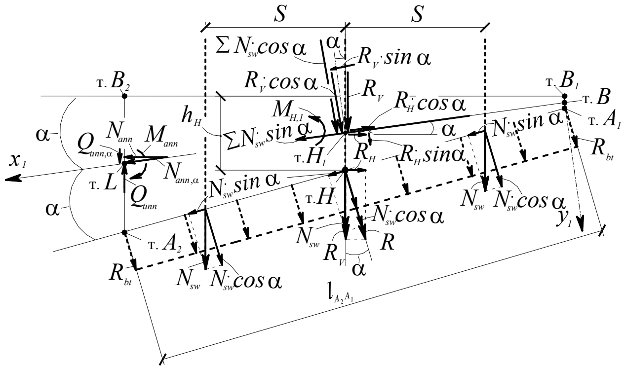
Рисунок 2 – Расчетной схеме клина для определения дополнительного поля напряженно-деформированного состояния в сечении 2-2
