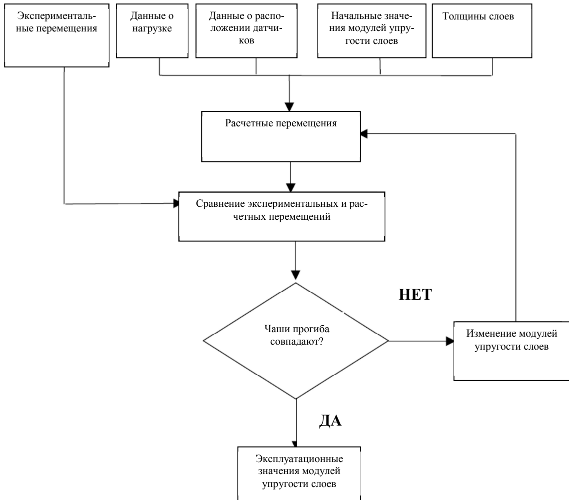
Рисунок 2 – Алгоритм определения модулей упругости слоев эксплуатируемых нежестких дорожных конструкций на стадии эксплуатации
