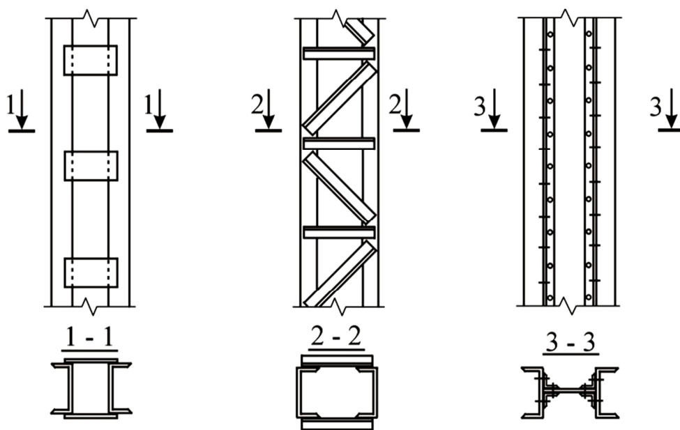
Рисунок 1 – Типы составных металлических колонн
