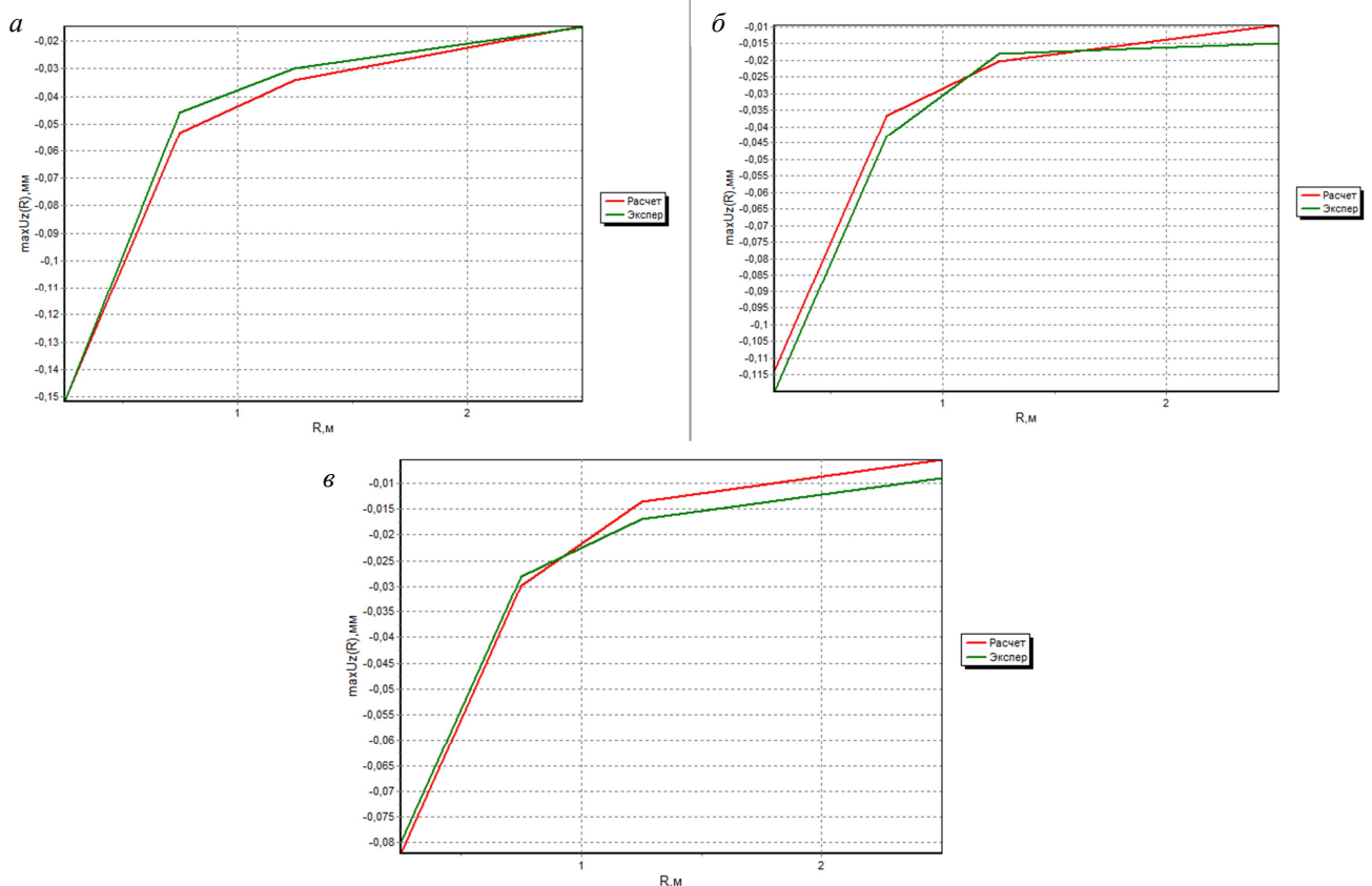
Рисунок 5 – Сопоставление экспериментальных чаш динамических прогибов и расчетных чаш, полученных с использованием комплекса «Vibrolab» а – расчетная и экспериментальная чаши прогибов на поверхности слоя песка; б – расчетная и экспериментальная чаши прогибов на поверхности слоя щебеночного основания; в – расчетная и экспериментальная чаши прогибов на поверхности слоя тощеого бетона
