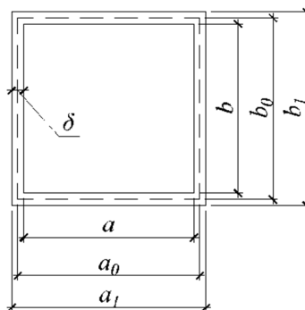
Рисунок 1 – Труба в виде прямоугольника
