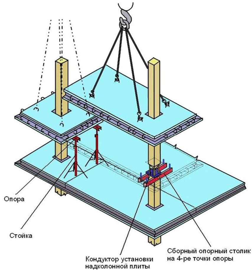
Рисунок 7 – Схема монтажа плит перекрытия в строительной системе КУБ-3V
