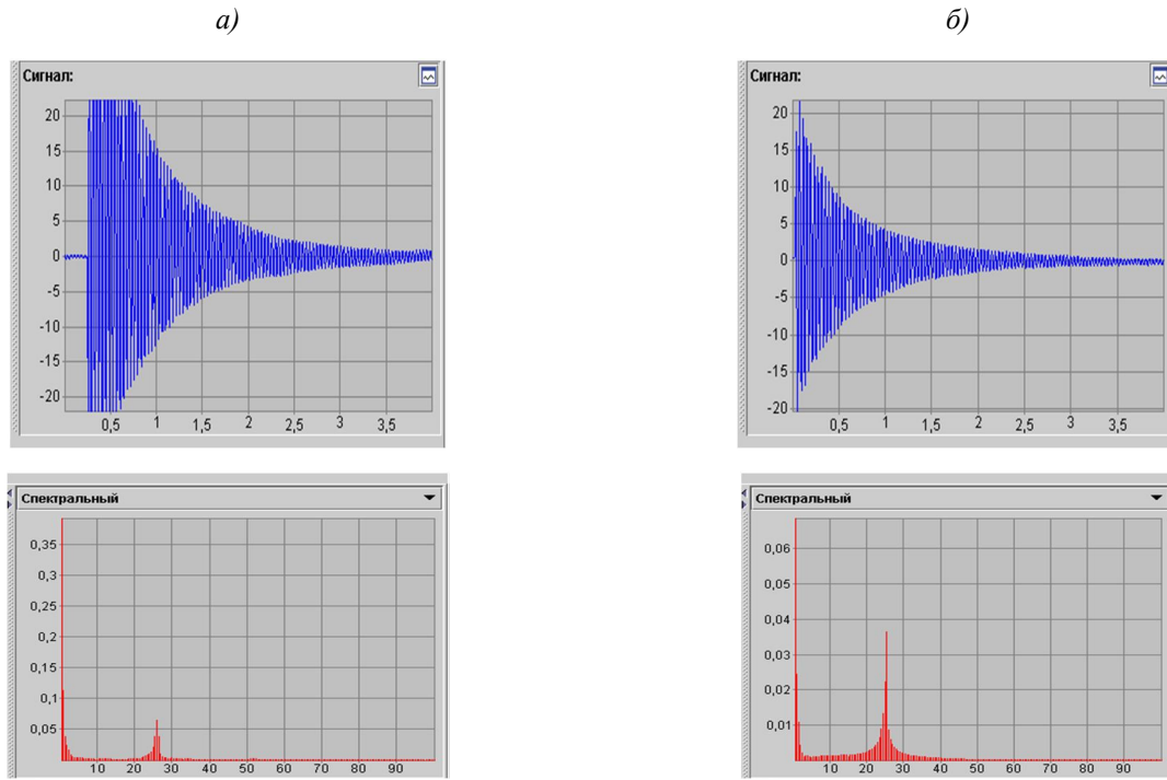
Рисунок 1 – Виброграммы и спектрограммы свободных поперечных колебаний железобетонных балок Б-2-1 и Б-6-1: а – балка Б-2-1; б – балка Б-6-1
