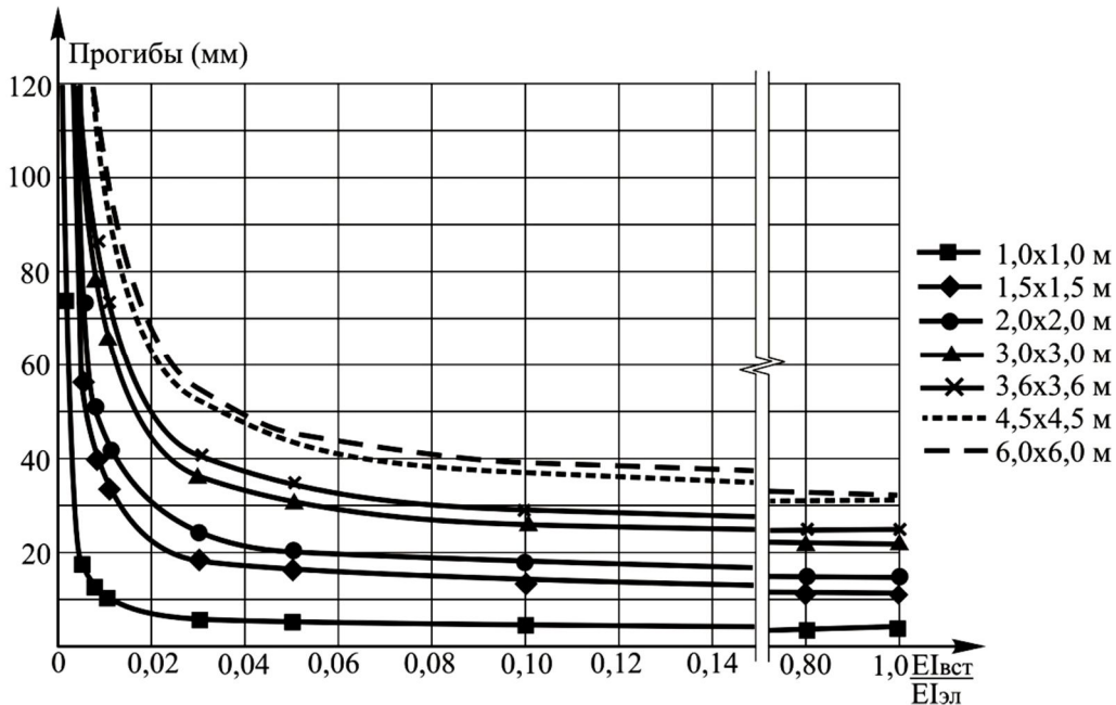
Рисунок 4 – Изменение прогибов в зависимости от соотношения жесткости вставки к жесткости элемента
