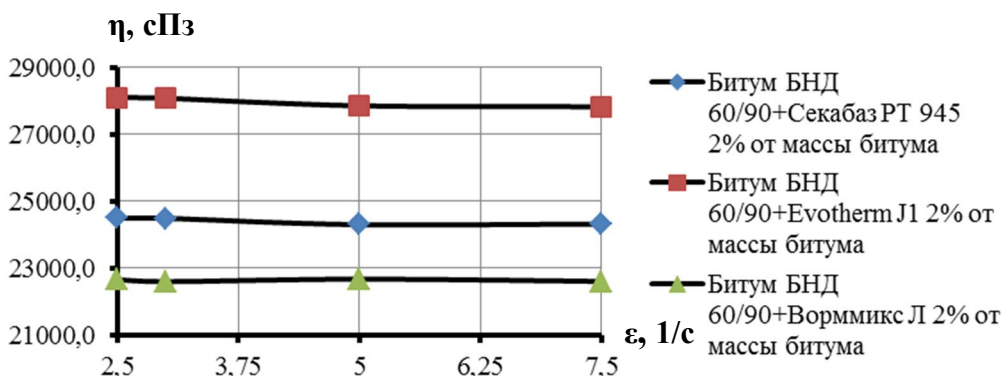
Рисунок 8 – Зависимость динамической вязкости \eta битума БНД 60/90 с добавками от скорости сдвига \epsilon при температуре 80^{\circ}\text{C}
