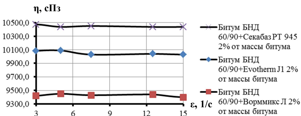
Рисунок 7 – Зависимость динамической вязкости \eta битума БНД 60/90 с добавками от скорости сдвига \epsilon при температуре 90^{\circ}\text{C}
