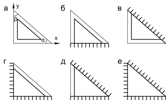
Рисунок 2 – Варианты граничных условий для пластинок в виде прямоугольных треугольников
