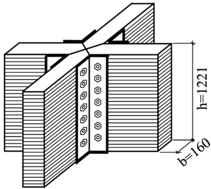
Рисунок 1 – Узел примыкания элементов
