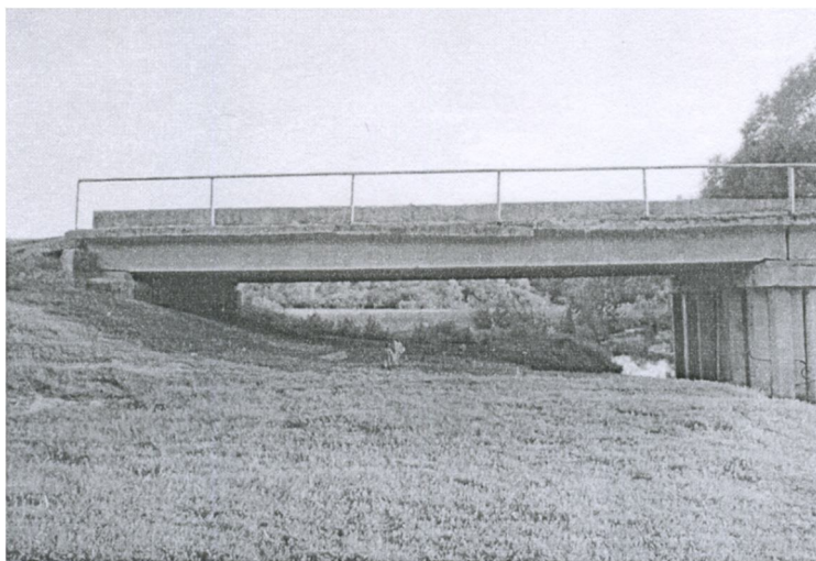
Рисунок 1 – Разрезной железобетонный мост через р. Рогозна в д. Старково Курской области
