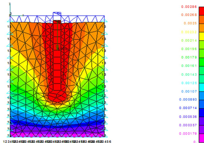
Рисунок 6 – Конечно-элементная модель буронабивной сваи с уширением и изополя перемещений от действия вертикальной нагрузки
