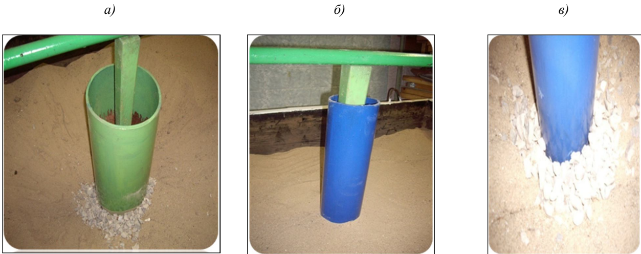
Рисунок 1 – Иллюстрации испытаний штампа в обсадных трубах в грунтовой лотке: а – диаметр трубы 300 мм со щебнем; б – диаметр трубы 200 мм без щебня в – диаметр трубы 200 мм со щебнем
