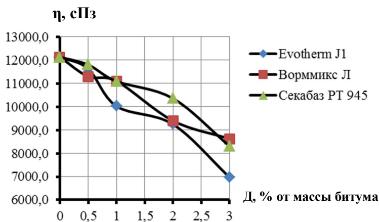
Рисунок 6 – Зависимость динамической вязкости \eta битума с добавками от их количества D при температуре 90^{\circ}\text{C}
