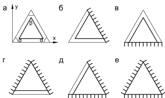
Рисунок 1 – Варианты граничных условий для пластинок в виде равнобедренных треугольников
