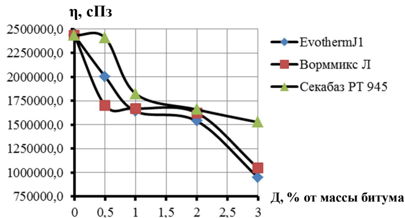
Рисунок 10 – Зависимость динамической вязкости \eta битума с добавками от их количества D при температуре 50°C
