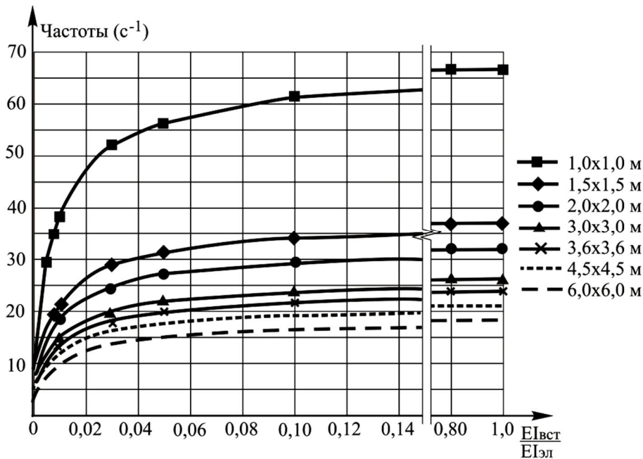
Рисунок 3 – Изменение частот собственных колебаний в зависимости от соотношения жесткости вставки к жесткости элемента
