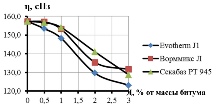
Рисунок 4 – Зависимость динамической вязкости \eta битума с добавками от их количества D при температуре 160°C
