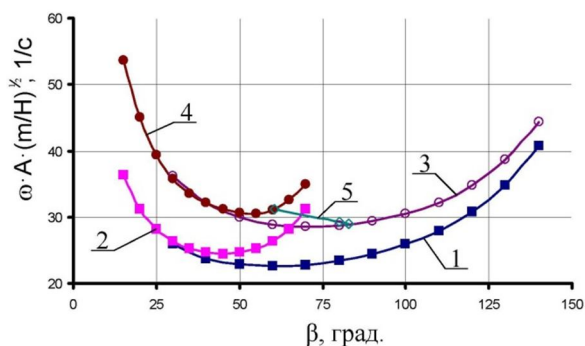
Рисунок 3 – Графики функций \omega - \beta
