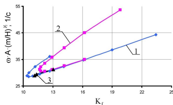
Рисунок 4 – Графики функций \omega - K_f
