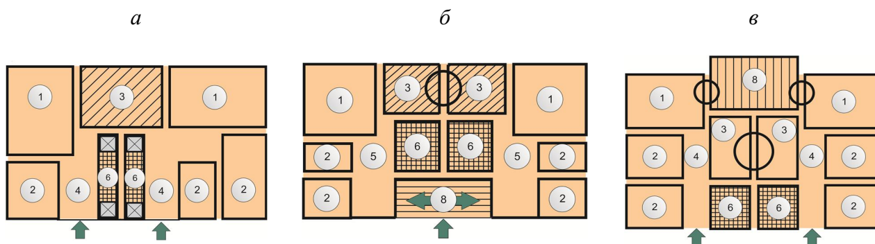
Рисунок 4 – Схемы жилых домов сложной структуры, состоящих из двух квартир с помещениями общего пользования: а – схема двух квартир с общей кухней-столовой; б – схема двух квартир с общей прихожей-верандой; в – схема двух квартир с общими летними помещениями (веранды) 1 – общая комната; 2 – спальня; 3 – кухня; 4 – прихожая; 5 – холл; 6 – санузел; 7 – кладовая; 8 – веранда
