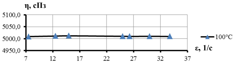
Рисунок 3 – Зависимость динамической вязкости \eta битума БНД 60/90 от скорости сдвига \epsilon при температуре 100°C
