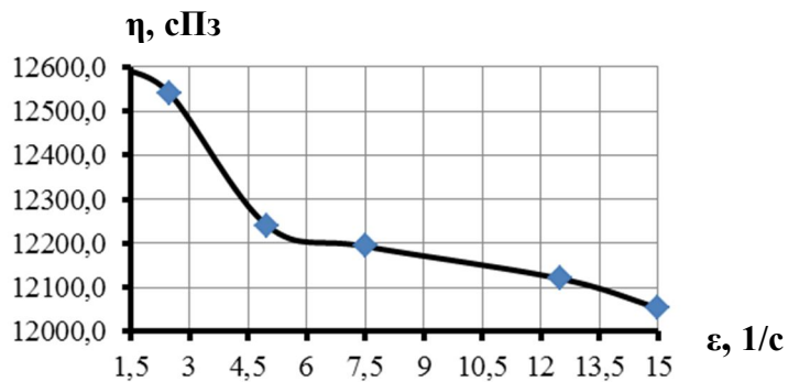
Рисунок 5 – Зависимость динамической вязкости \eta битума БНД 60/90 от скорости сдвига \epsilon при температуре 90°C
