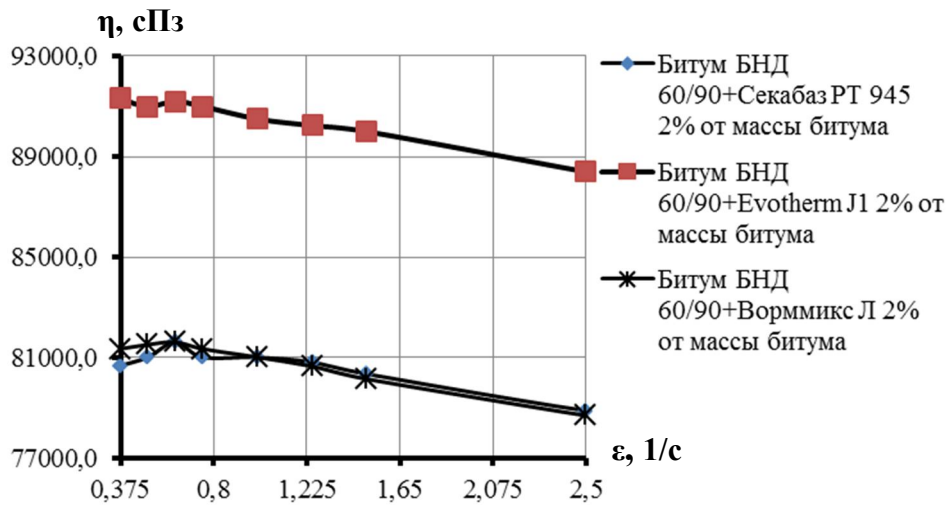
Рисунок 9 – Зависимость динамической вязкости \eta битума БНД 60/90 с добавками от скорости сдвига \epsilon при температуре 70°C
