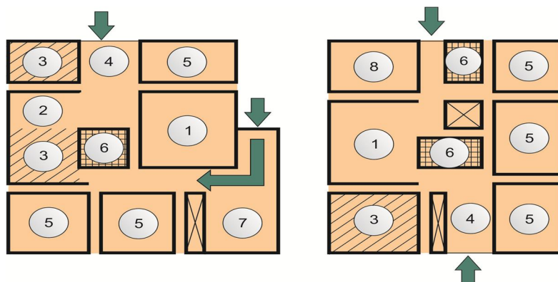
Рисунок 2 – Схемы квартир с расширенным составом жилых и подсобных помещений, квартиры с дополнительным входом: 1 – общая комната; 2 – столовая; 3 – кухня; 4 – прихожая; 5 – спальня; 6 – санузел; 7 – веранда; 8 – хозяйственная комната
