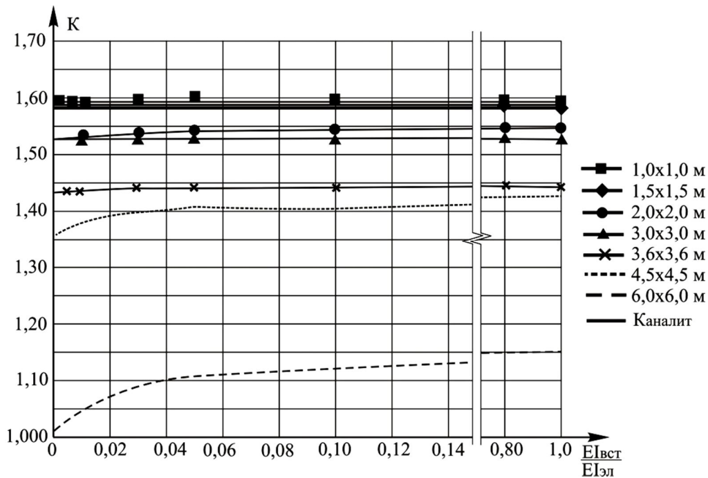
Рисунок 5 – Изменение коэффициента K_{расч} в зависимости от соотношения жесткости вставки к жесткости элемента
