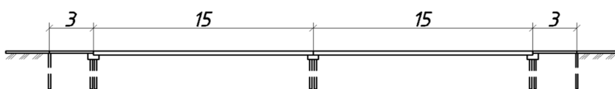
Рисунок 2 – Расчетная схема моста
