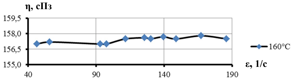
Рисунок 2 – Зависимость динамической вязкости \eta битума БНД 60/90 от скорости сдвига \epsilon при температуре 160°C
