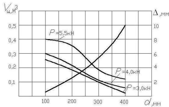
Рисунок 5 – График зависимости осадки буронабивной сваи от объема щебня, диаметра обсадной трубы и нагрузки
